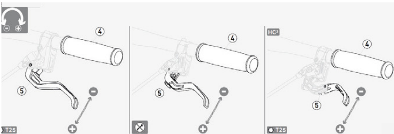
112. ábra: MAGURA tárcsafék fékkar markolatszélességének beállítása
