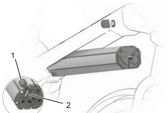
53. ábra: Beépített akkumulátor feltöltési szintjelző elhelyezkedése
