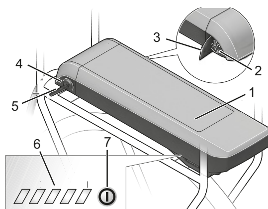
35. ábra: Csomagtartó-akkumulátor részlet
