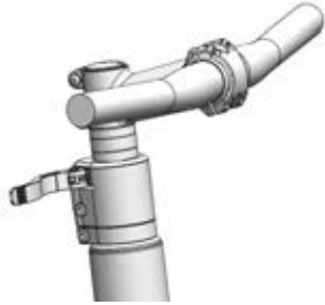
143. ábra: Példa: All Up nyitott kormányzár gyorskioldóval
