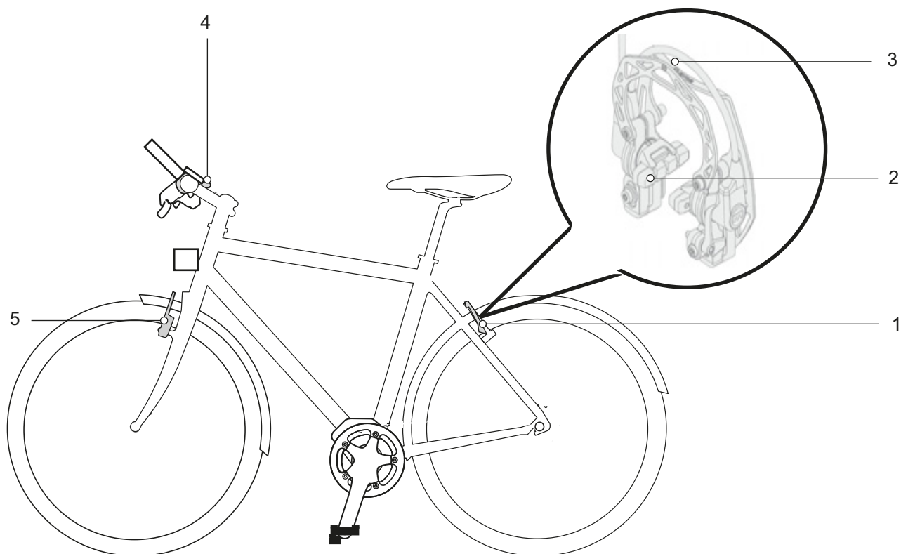
23. ábra: Fékrendszer felnifékkal részlet, példa: MAGURA HS22
