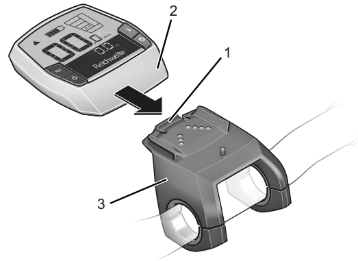
137. ábra: A fedélzeti számítógép hátracolása (2) a fedélzeti számítógép rögzítésével (1) a tartó ütközőjéig (3)
