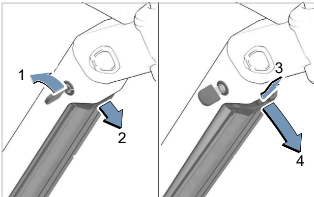
201. ábra: Beépített akkumulátor kiszerezése
