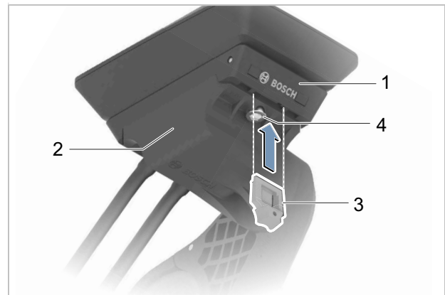
177. ábra: A vezérlőegység-csavar elhelyezkedése
