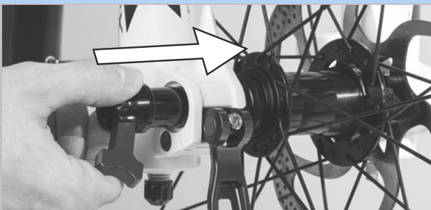
120. ábra: A keresztteget betolása nyírányban
