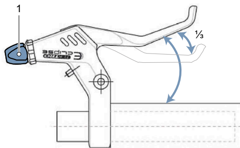
243. ábra: Fordítsa el az állítócsavart (1), amíg a fékek a kézifék 1/3-nyi mozgása után be nem kapcsolódnak
