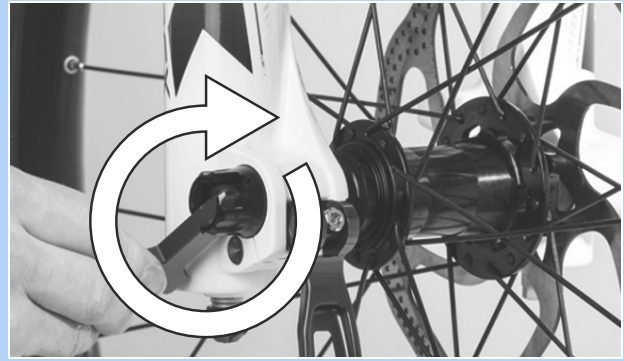
121. ábra: A teget meghúzása nyírányban
