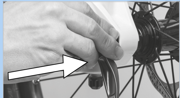
127. ábra: A gyorsár betolása nyílrányban
