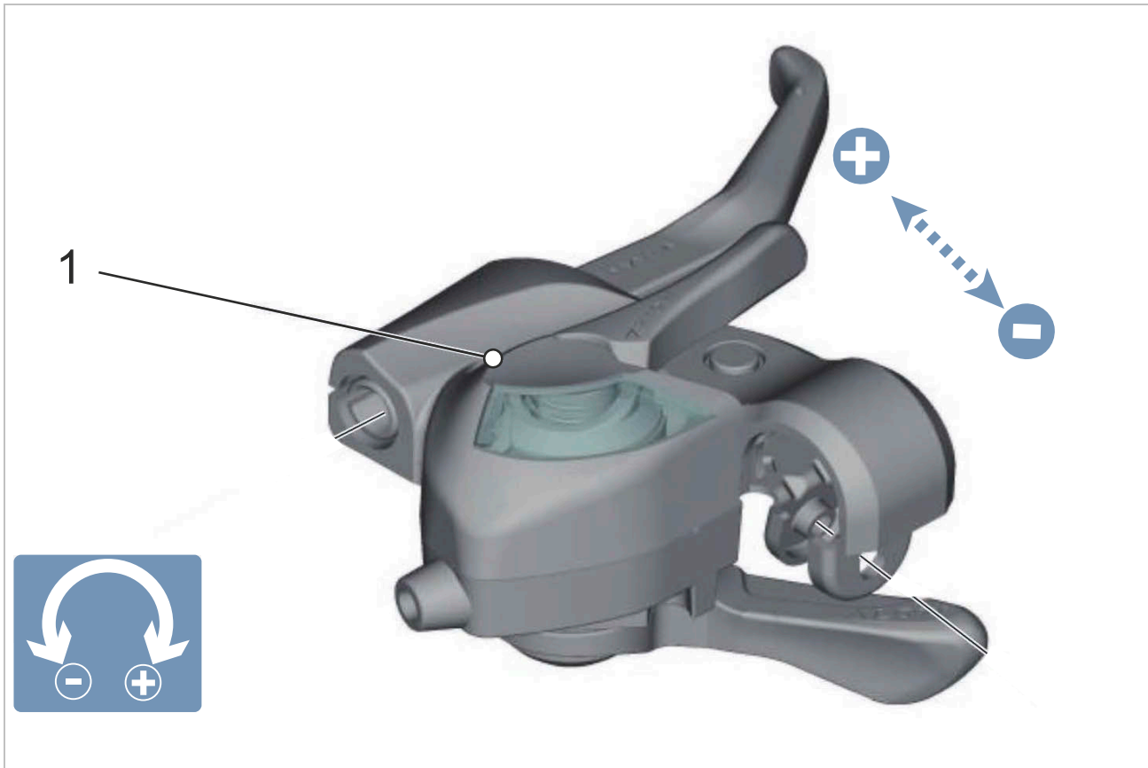
166. ábra: Állítócsavar (1) helyzete
