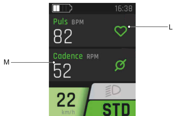
92. ábra: Fitness FŐKIJELZÉS áttekintése
