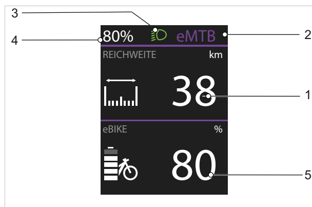
76. ábra: RANGE KÉPERNYŐ áttekintése, 1. oldal
