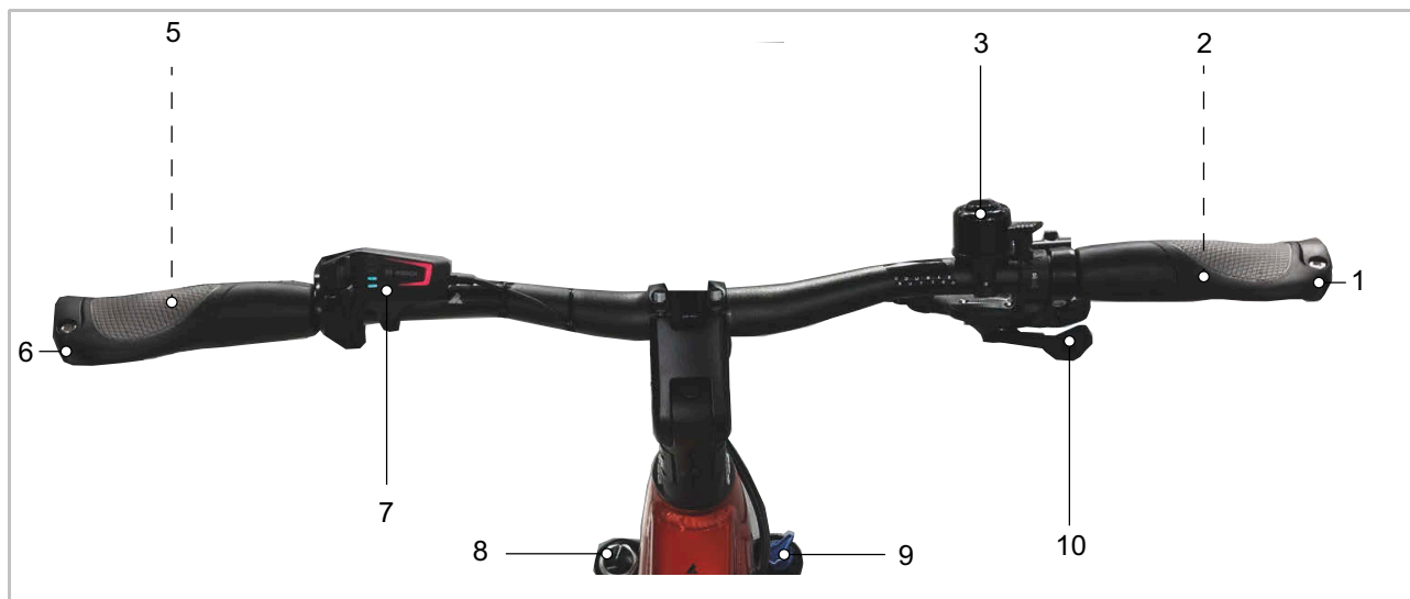
63. ábra: BOSCH LED Remote fedélzeti számítógéppel felszerelt kormány részletes nézete, példa
