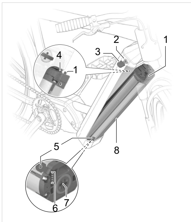
54. ábra: A PowerTube akkumulátor részletei
