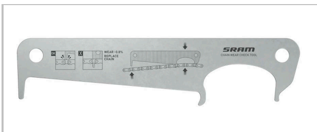
247. ábra: SRAM mérőidom példája
