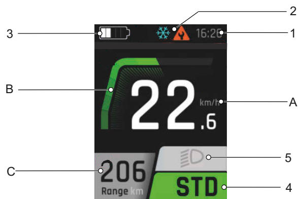
87. ábra: Drive FŐKIJELZÉS áttekintése
