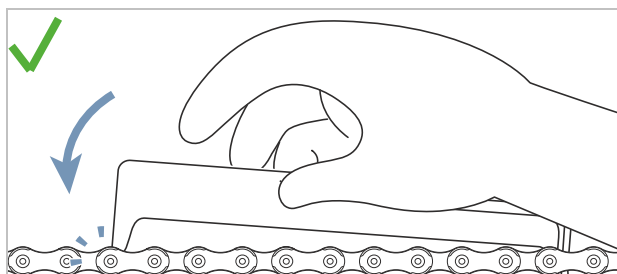
252. ábra: A mérőidom nem illeszkedik
