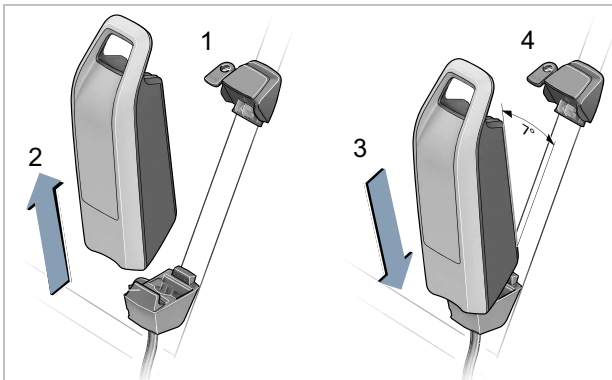
203. ábra: Vázakkumulátor kiszerelése és beszerelése
