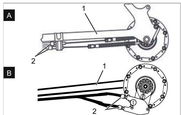
Illustration 222 : Douilles de réglage (2) sur deux modèles alternatifs (A et B) d'un changement de vitesse actionné par câble à deux câbles sur la base de cadre (1)
