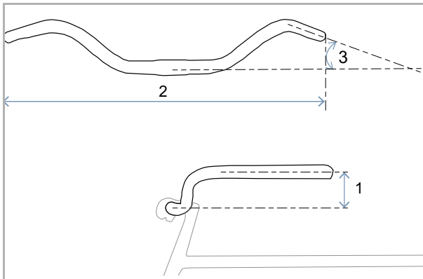
Illustration 13 : Dimensions du guidon
