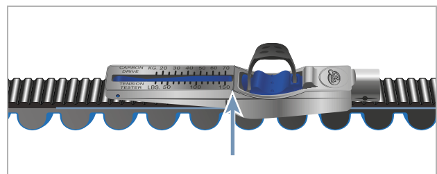
Illustration 212 : Gabarit de contrôle sur la courroie
