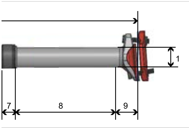
Illustration 78 : Dimensions de la tige de selle LIMOTEC, A1
