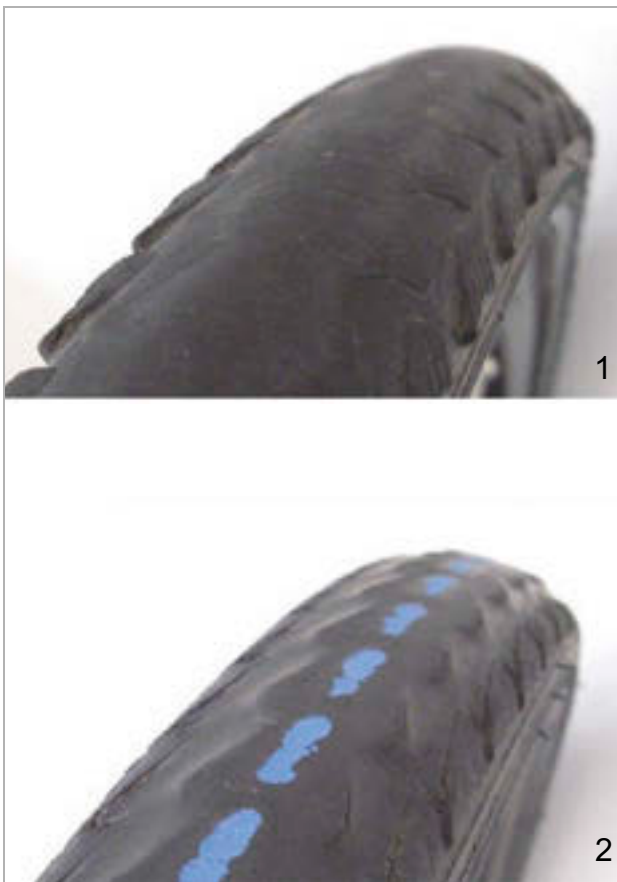
Illustration 194 : Pneu sans profil pouvant être changé (1) et pneu avec protection anti-crevaison visible (2) devant être changé
