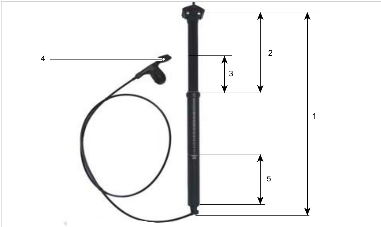
Illustration 47 : Structure et dimensions de la tige de selle A3
