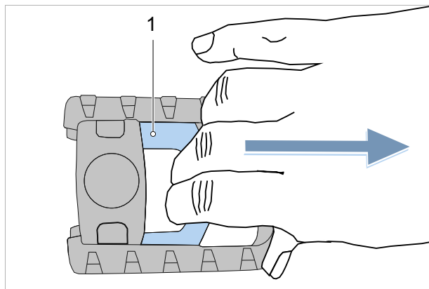
Illustration 189 : Tirer le verrou de pliage de la pédale (1) vers le bas
