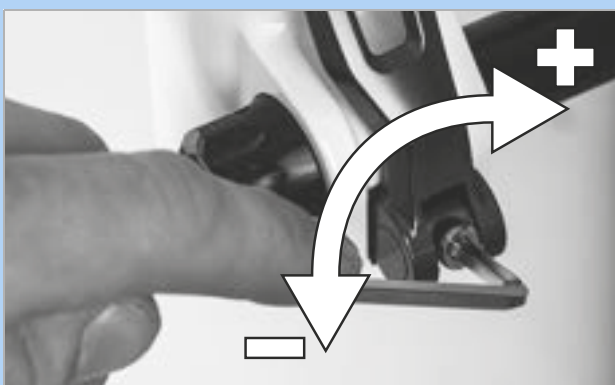
Illustration 93 : Régler la force de serrage de l'attache rapide
