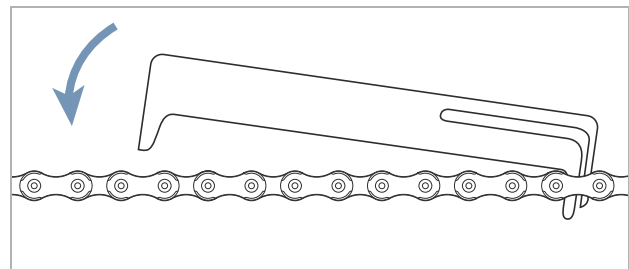
Illustration 204 : Abaisser le gabarit de mesure à gauche
