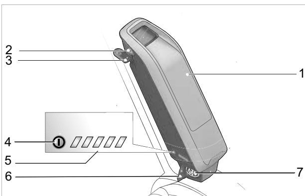
Illustration 60 : Détail d'une batterie sur cadre
