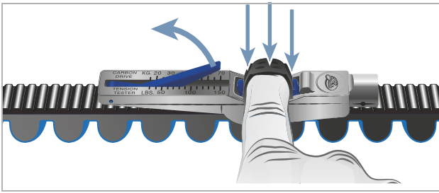
Illustration 213 : Abaisser le gabarit de contrôle avec un doigt
