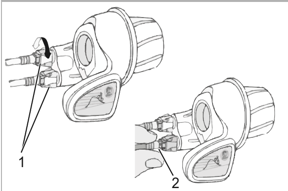
Illustration 223 : Poignée de vitesse rotative avec douilles de réglage (1) avec jeu de rotation (2)
