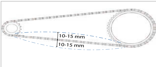
Illustration 219 : Exemple de contrôle de la tension de la chaîne : 5 mm vers le haut, 10 mm vers le bas = écart de 15 mm
