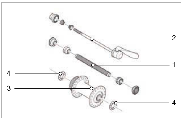
Illustration 38 : Exemple d'un moyeu de roue avant, SHIMANO
