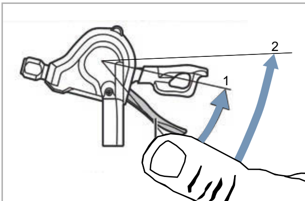
Illustration 183 : Changement de vitesse avec manette A, exemple d'un changement de vitesse SL-M5000
