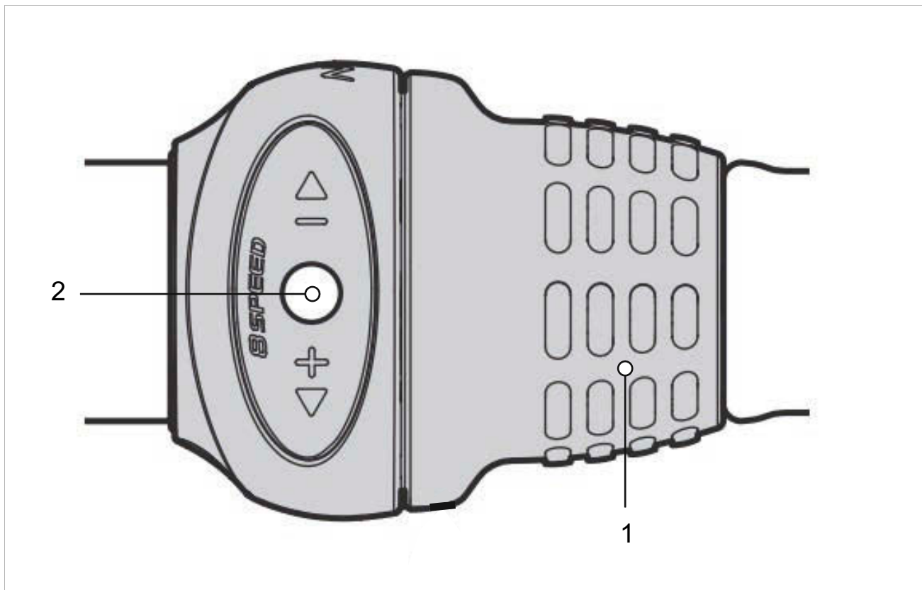
Illustration 69 : Poignée de vitesse rotative SHIMANO SL-C30000-7, vue de dessus
