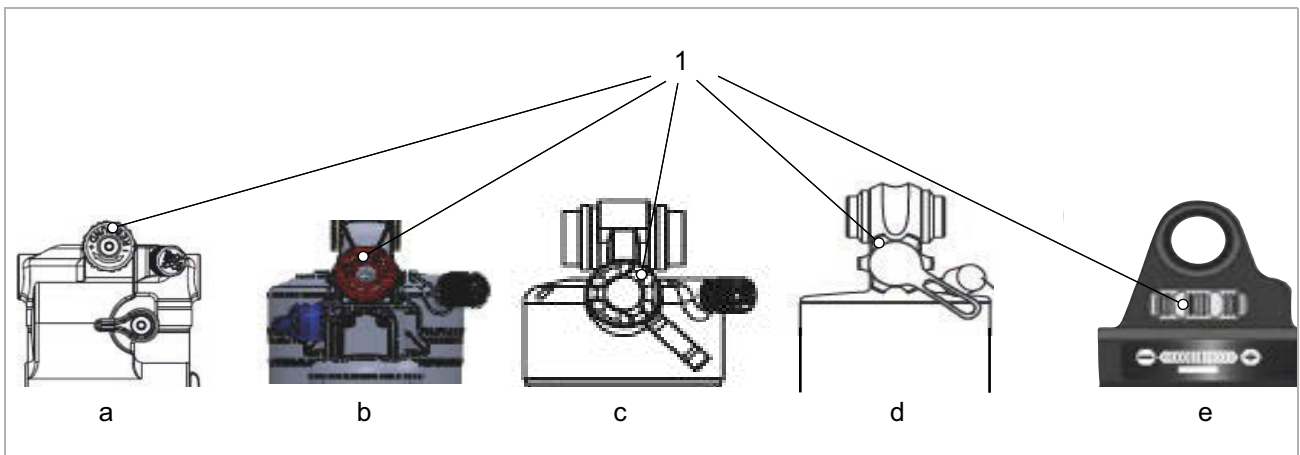
Illustration 237 : Position de la molette de détente SR Suntour sur amortisseur arrière Triair2 (a), Triair (b), EDGE-comp (c), EDGE (d) et RAIDON (e)
