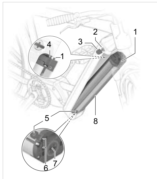
Illustration 58 : Détails PowerTube
