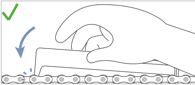
Illustration 205 : Le gabarit de mesure ne passe pas
