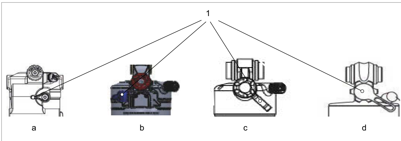
Illustration 241 : Position du levier de compression SR Suntour sur amortisseur arrière Triair2 (a), Triair (b), EDGE-comp (c), EDGE (d)
