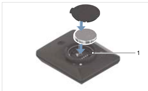
Illustration 151 : Insérer la pile en veillant à la position du joint (1)
