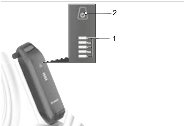
Illustration 74 : Éléments d'affichage et de commande de la batterie BOSCH PowerPack
