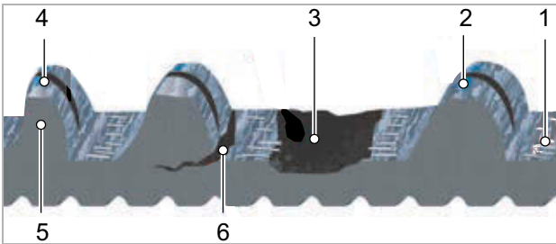
Illustration 207 : Signes d'usure d'une courroie
