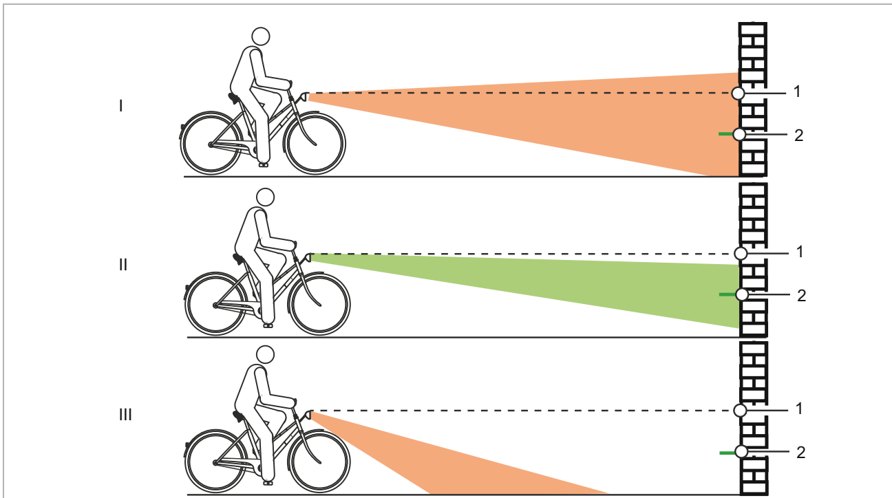
Illustration 218 : Feu réglé trop haut (1), correctement (2) et trop bas (3)
