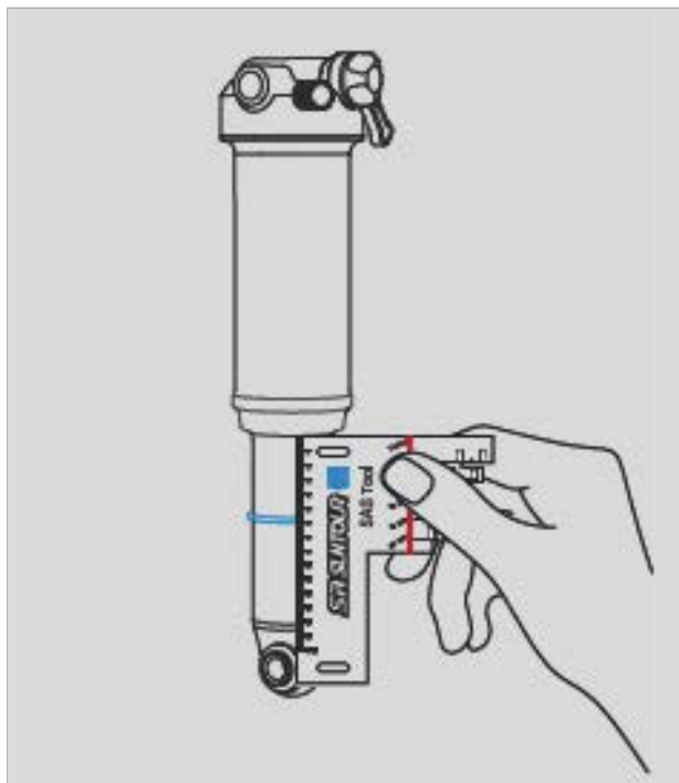
Illustration 142 : Mesurer la course de suspension totale
