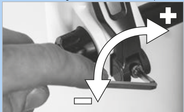
Illustration 225 : Régler la force de serrage de l'attache rapide
