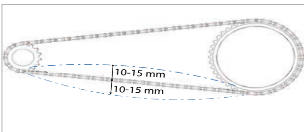
Illustration 197 : Exemple de contrôle de la tension de la chaîne : 5 mm vers le haut, 10 mm vers le bas = écart de 15 mm
