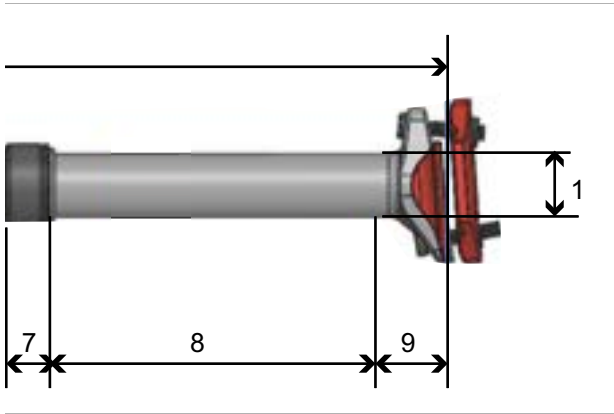
Illustration 79 : Dimensions de la tige de selle LIMOTEC, A1L
