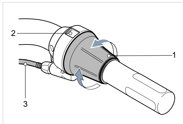
Illustration 185 : Changement de vitesse SHIMANO SL-C30000-70
