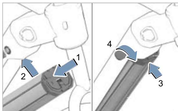
Illustration 171 : Insérer la batterie intégrée
