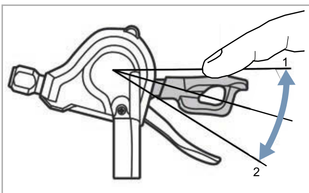
Illustration 184 : Changement de vitesse avec manette B, exemple d'un changement de vitesse SL-M5000
