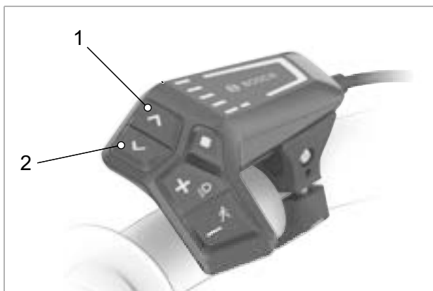
Illustration 177 : Position de la touche d'augmentation de la luminosité (2) et de la touche de réduction de la luminosité (1)
