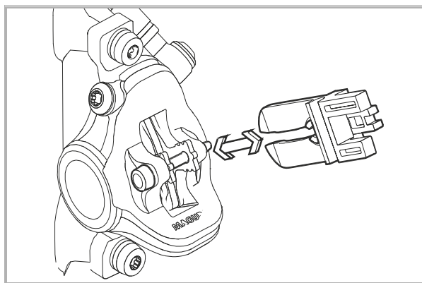
Illustration 82 : Insérer la cale de transport
