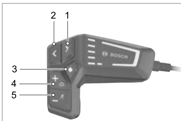
Illustration 155 : Éléments de commande BOSCH LED Remote
