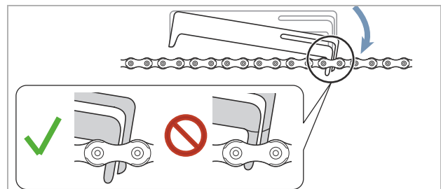
Illustration 203 : Le gabarit de mesure s'insère
