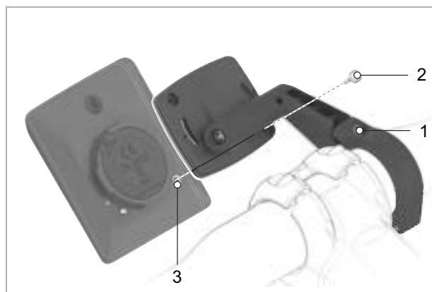
Illustration 154 : Position de la vis du jeu de direction
