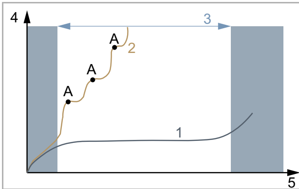
Illustration 190 : Diagramme d'usure, durée de service (x) par rapport à l'enlèvement de matière (y)
