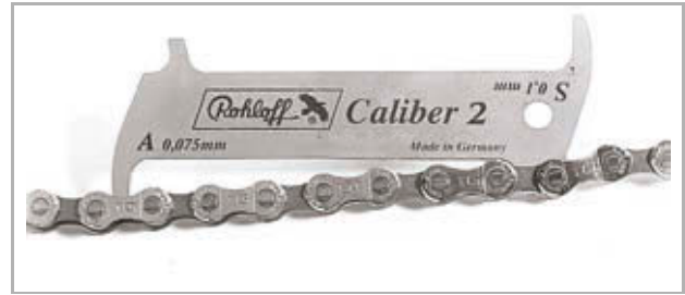
Illustration 201 : Exemple d'un gabarit de mesure ROHLOFF
