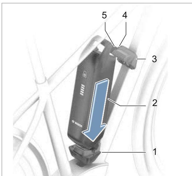
Illustration 172 : Insérer la batterie PowerPack
