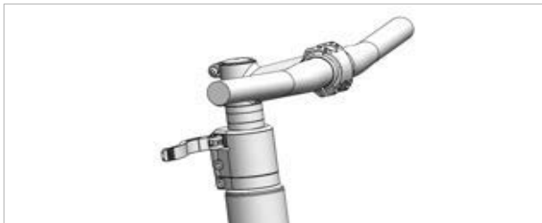
Illustration 186 : Exemple d'un All Up avec levier de serrage de la potence ouvert
