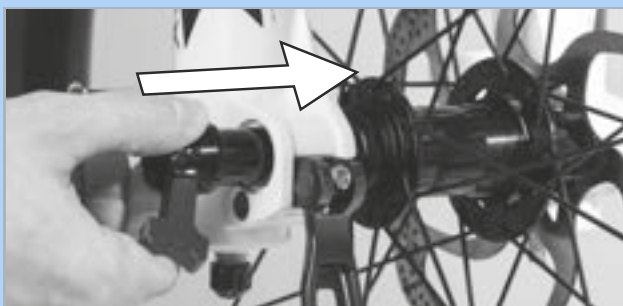
Illustration 88 : Enfoncez l'axe transversal dans le sens de la flèche
