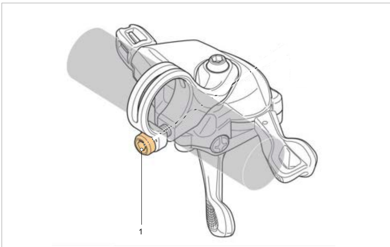
Illustration 133 : Position de la vis de fixation du levier de vitesse SHIMANO (1)
