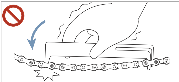
Illustration 206 : Le gabarit de mesure passe
