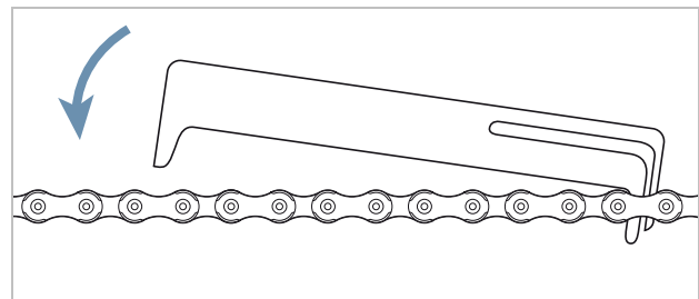
Illustration 148 : Abaisser le gabarit de mesure à gauche
