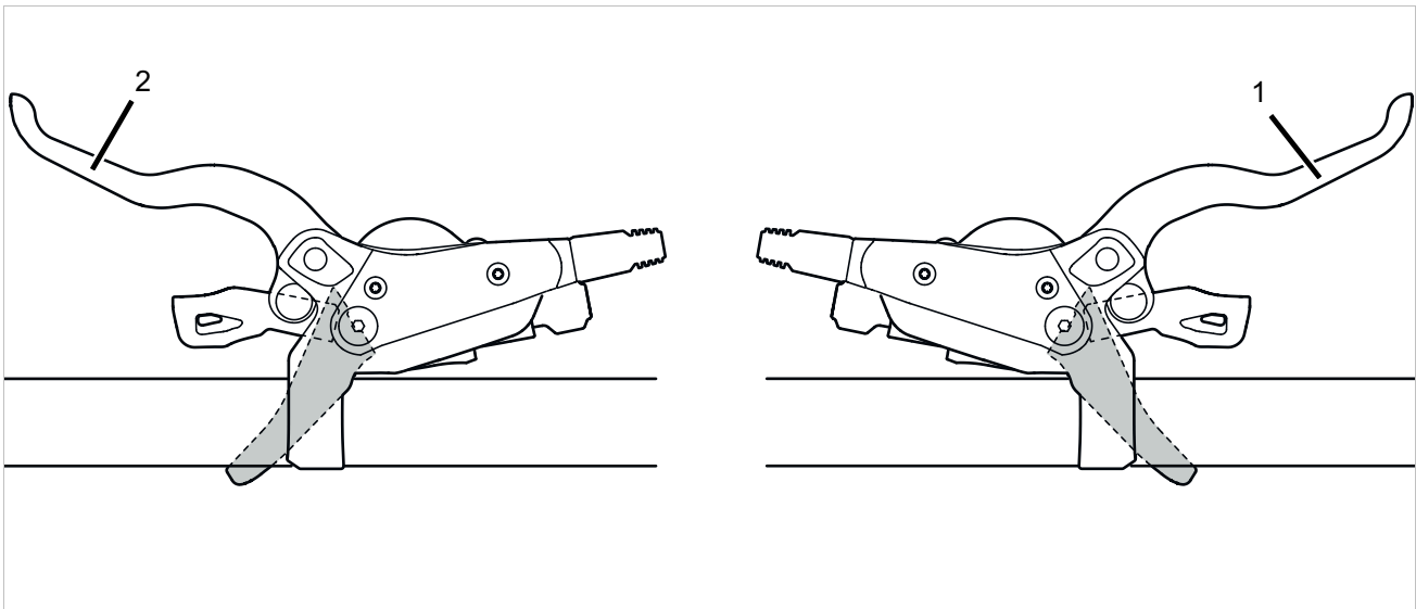
Illustration 45 : Freins à main arrière (1) et avant (2), exemple d'un frein SHIMANO
