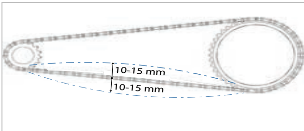
Illustration 163 : Exemple de contrôle de la tension de la chaîne : 5 mm vers le haut, 10 mm vers le bas = écart de 15 mm
