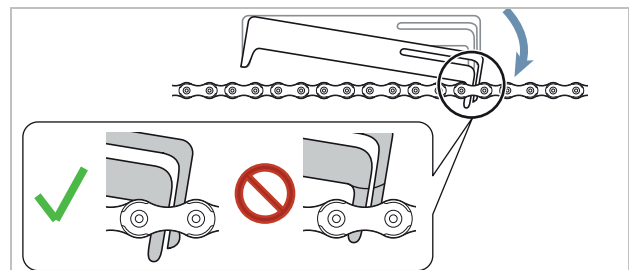
Illustration 147 : Le gabarit de mesure s'insère
