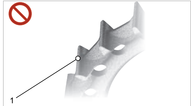
Illustration 153 : Profil de cran usé
