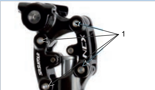
Illustration 170 : Points de lubrification de la tige de selle suspendue SR SUNTOUR
