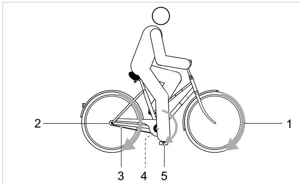
Illustration 38 : Schéma du système d'entraînement mécanique
