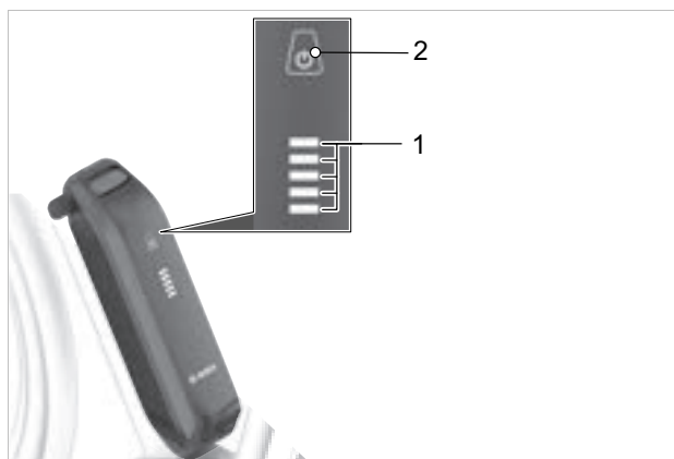
Illustration 48 : Éléments d'affichage et de commande de la batterie BOSCH PowerPack
