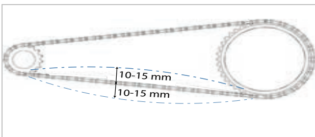
Illustration 141 : Exemple de contrôle de la tension de la chaîne : 5 mm vers le haut, 10 mm vers le bas = écart de 15 mm
