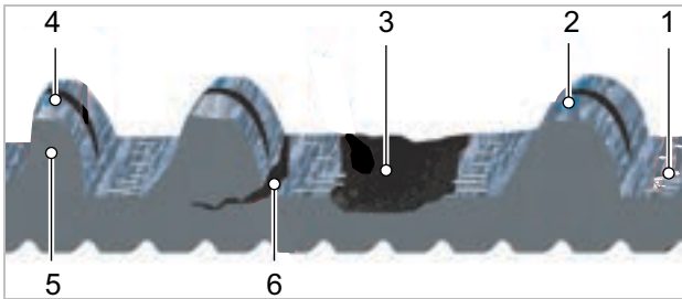
Illustration 151 : Signes d'usure d'une courroie
