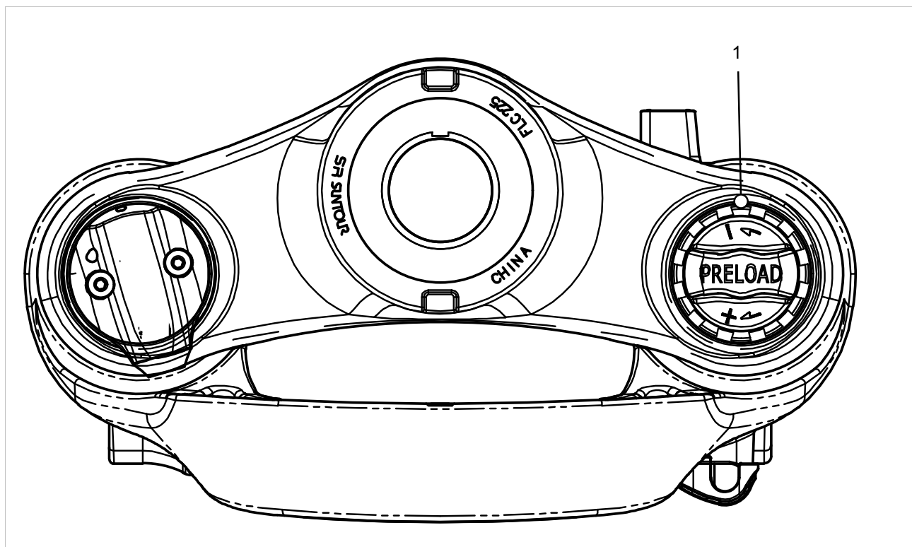
Illustration 107 : Exemple d'une SR SUNTOUR, molette de réglage du sag sur la couronne de fourche
