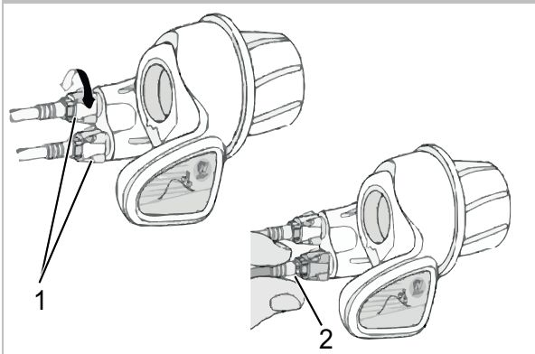
Illustration 167 : Poignée de vitesse rotative avec douilles de réglage (1) avec jeu de rotation (2)
