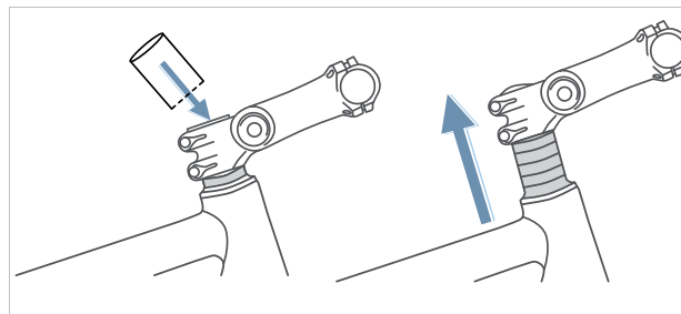
Illustration 92 : Relever la potence Ahead en montant une rondelle d'écartement
