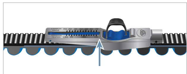
Illustration 156 : Gabarit de contrôle sur la courroie
