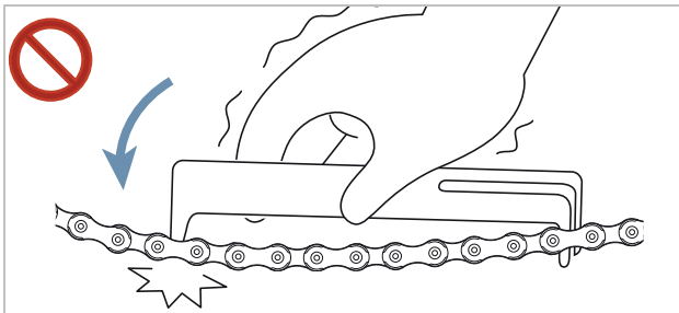
Illustration 150 : Le gabarit de mesure passe
