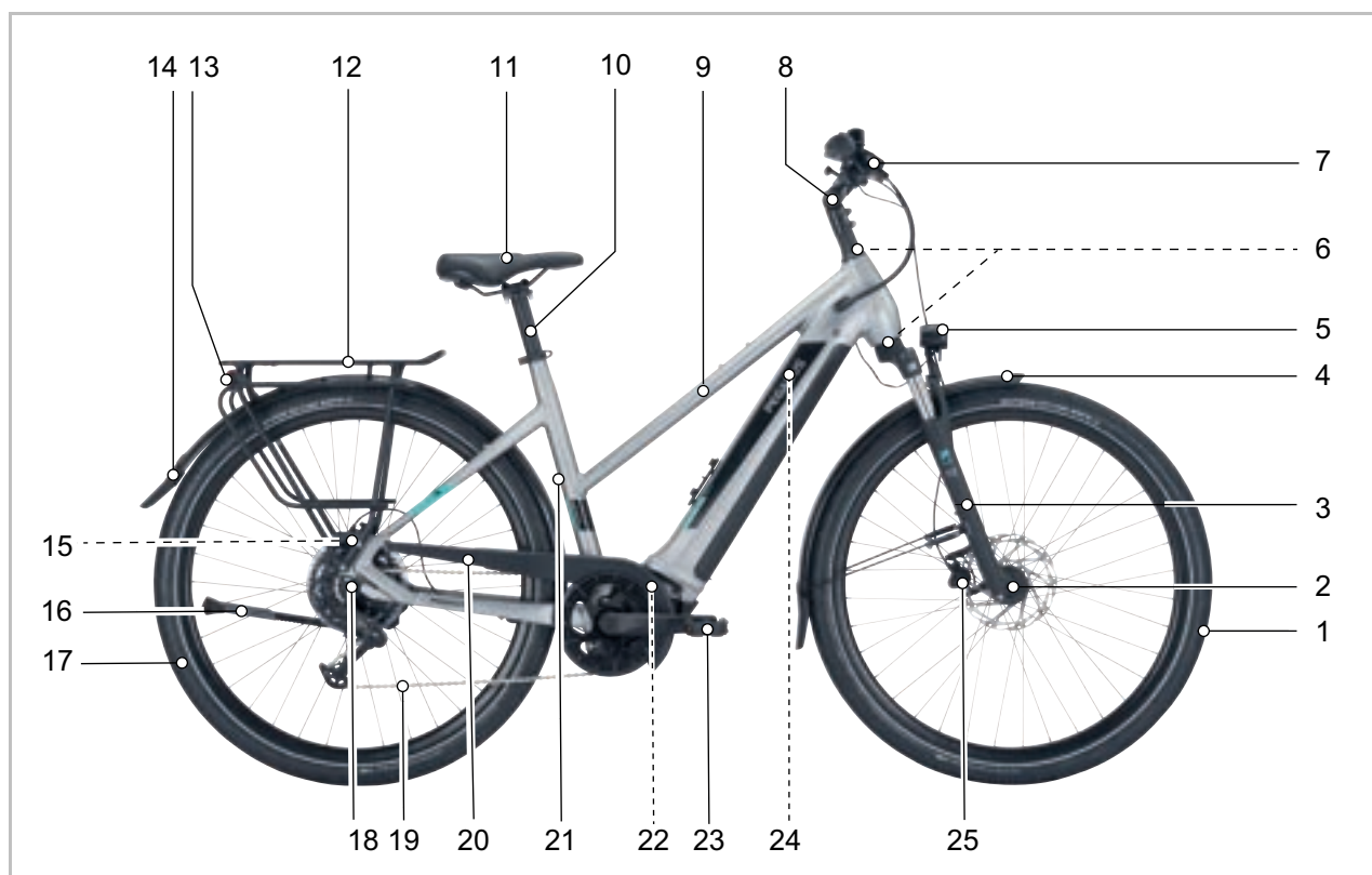
Illustration 3 : Vélo électrique vu de droite, exemple d'un Pegasus Evo CX
