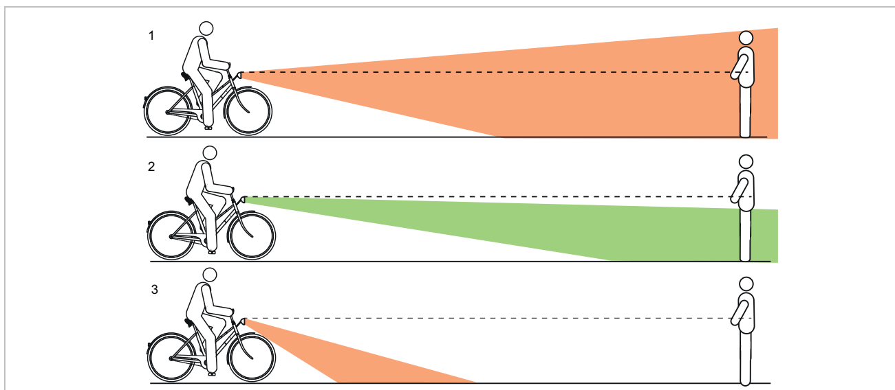
Illustration 108 : Feu réglé trop haut (1), correctement (2) et trop bas (3)
