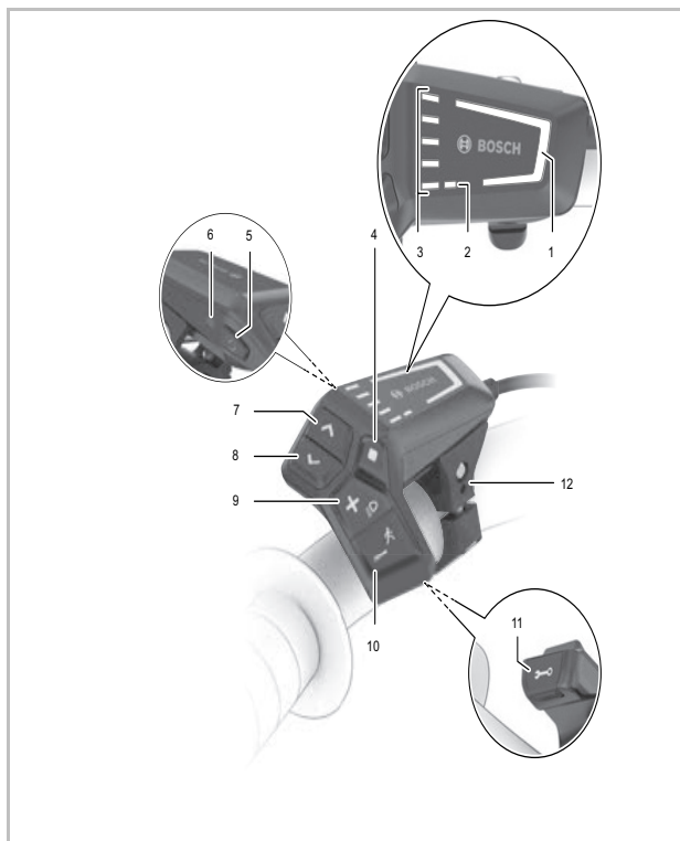
Illustration 123 : Aperçu de l'unité de commande BOSCH LED Remote
