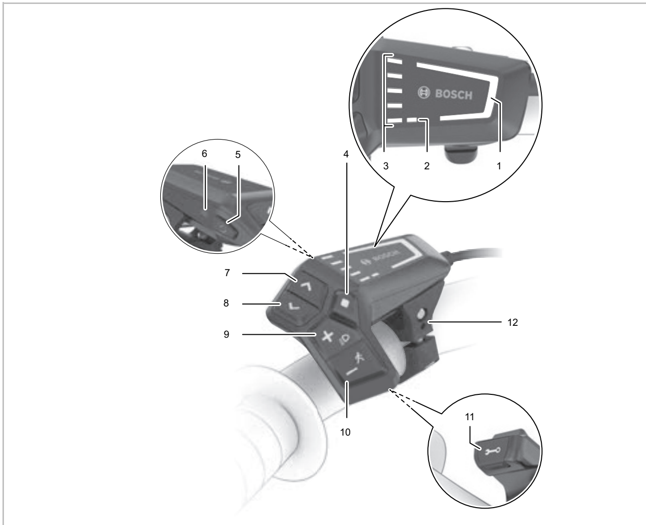
Illustration 44 : Aperçu de l'ordinateur de bord BOSCH LED Remote
