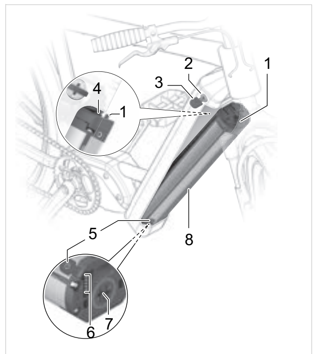
Illustration 43 : Détails PowerTube
