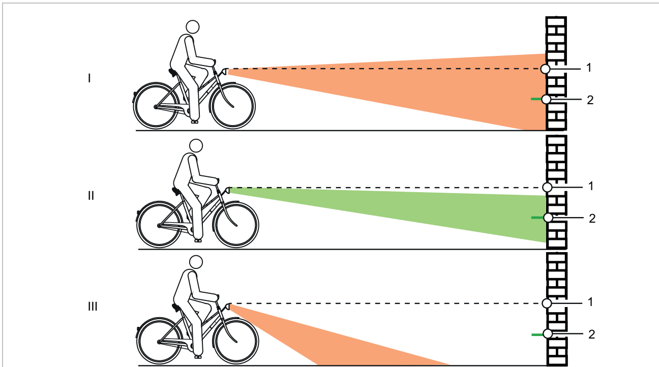
Illustration 162 : Feu réglé trop haut (1), correctement (2) et trop bas (3)
