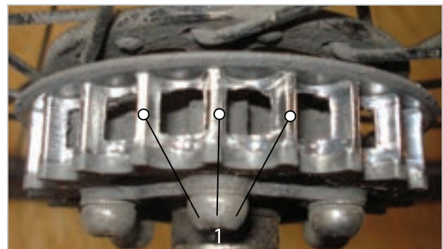
Illustration 154 : Exemple de photo d'un profil de cran usé
