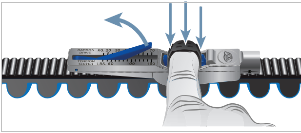
Illustration 157 : Abaisser le gabarit de contrôle avec un doigt
