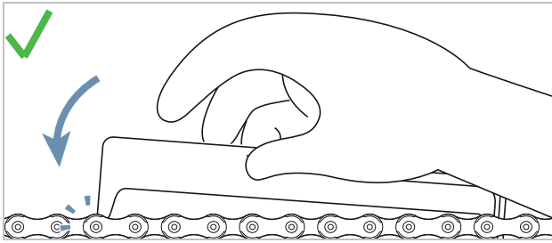
Illustration 149 : Le gabarit de mesure ne passe pas
