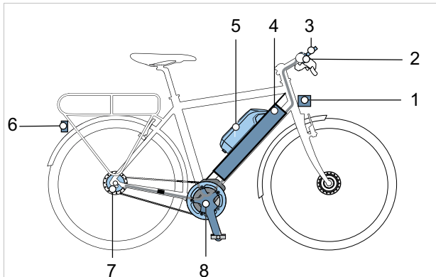
Illustration 41 : Schéma du système d'entraînement électrique avec composants électriques
