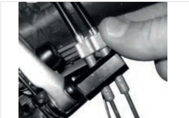
Illustration 164 : Sur les versions de moyeux ROHLOFF avec commande interne du changement de vitesse, le dispositif de réglage de la tension est situé sur le contre-support de tension.
