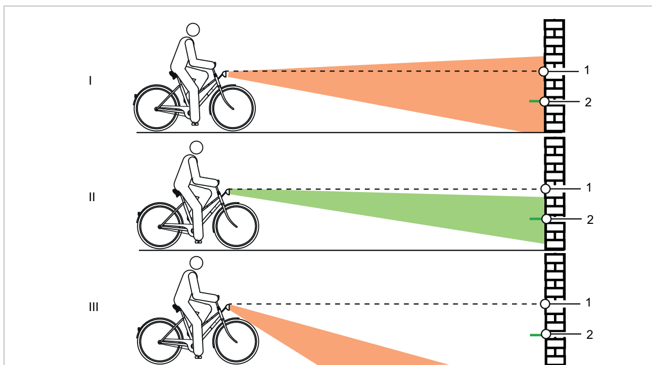
Illustration 110 : Feu réglé trop haut (1), correctement (2) et trop bas (3)
