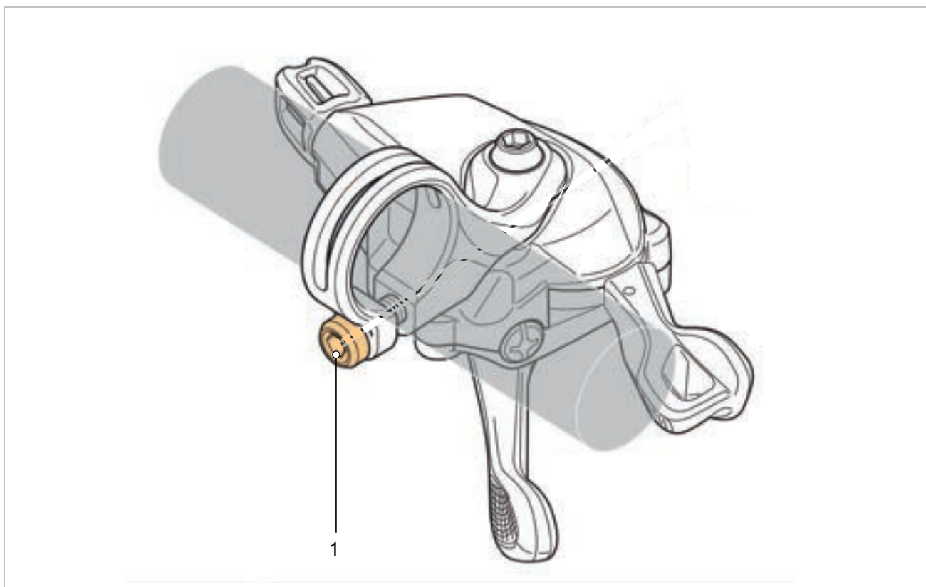
Illustration 103 : Position de la vis de fixation du levier de vitesse SHIMANO (1)
