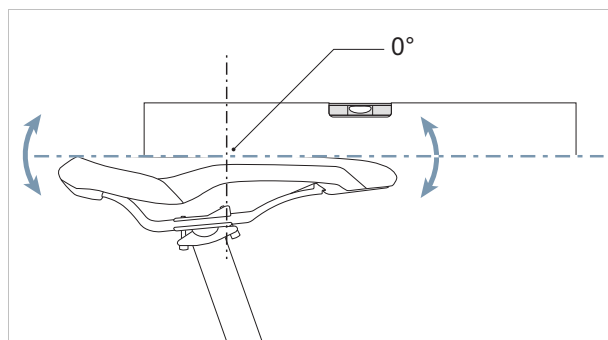
Illustration 86 : Inclinaison de la selle horizontale avec inclinaison de 0° au milieu de la selle
