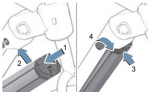
Illustration 121 : Insérer la batterie intégrée
