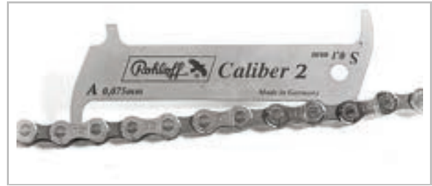
Illustration 145 : Exemple d'un gabarit de mesure ROHLOFF
