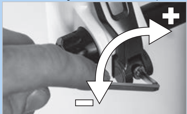
Illustration 169 : Régler la force de serrage de l'attache rapide
