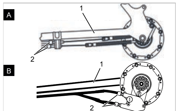
Illustration 166 : Douilles de réglage (2) sur deux modèles alternatifs (A et B) d'un changement de vitesse actionné par câble à deux câbles sur la base de cadre (1)
