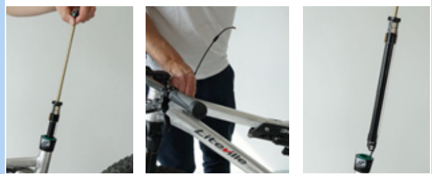
Figura 146: Estrazione della cartuccia
