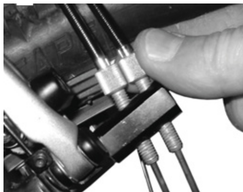
Figura 134: Le versioni del mozzo Rohloff con comando interno del cambio hanno i regolatori del tensionamento sul controsupporto di tensionamento
