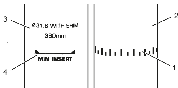
Figura 73: Particolare dei cannotti reggisella, esempi di segno indicante la minima profondità di inserimento
