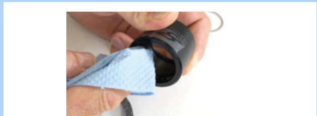
Figura 154: Pulizia della boccola esterna
