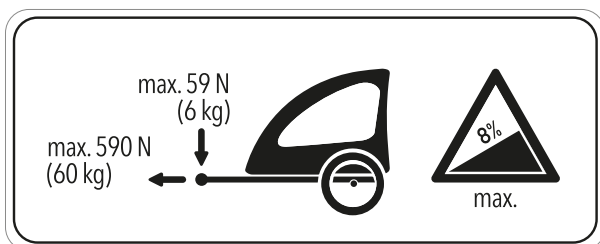
Figura 102: Cartello di avviso rimorchio
