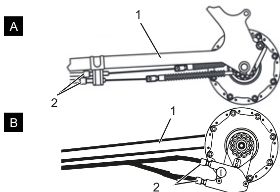
Figura 137: Bocche di regolazione (2) di due versioni alternative (A e B) di un cambio azionato da cavo doppio sul fodero orizzontale (1)
