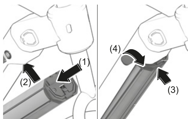
Figura 110: Montaggio della batteria integrata
