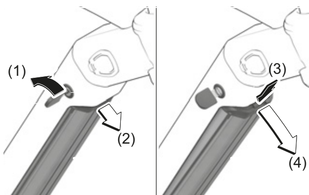
Figura 109: Smontaggio della batteria integrata
