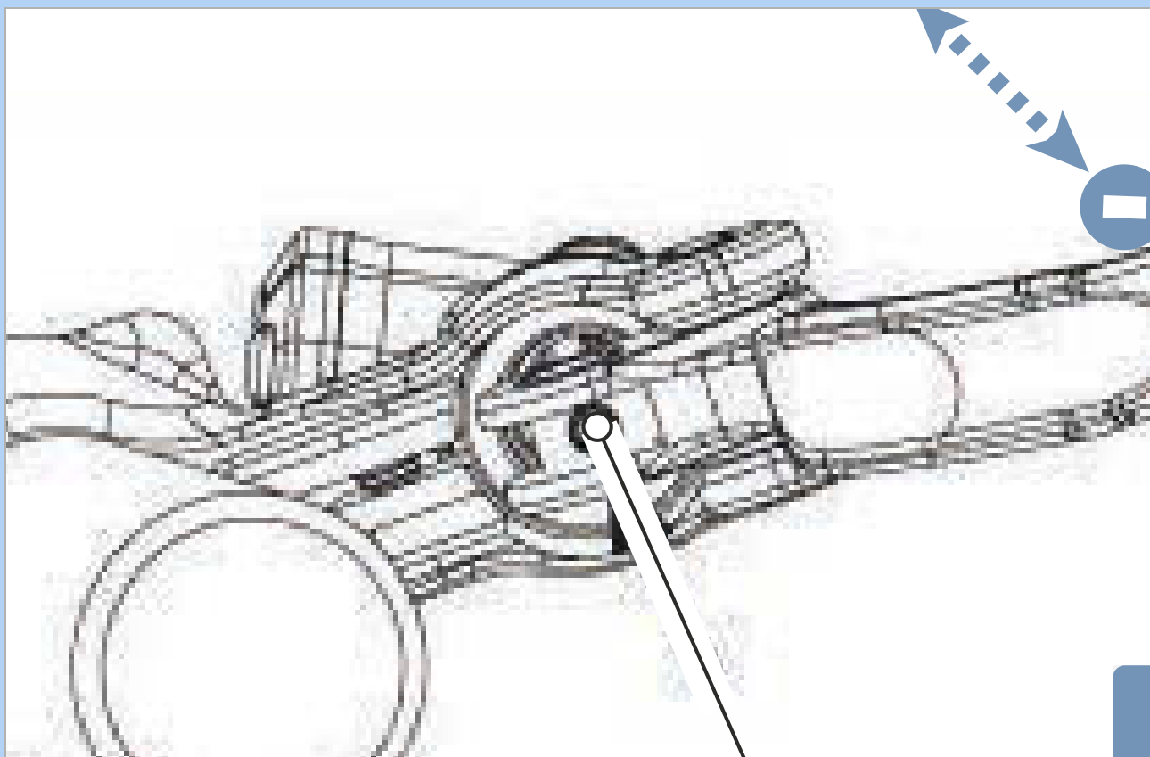
Figura 134: Posizione della vite di regolazione (1)
