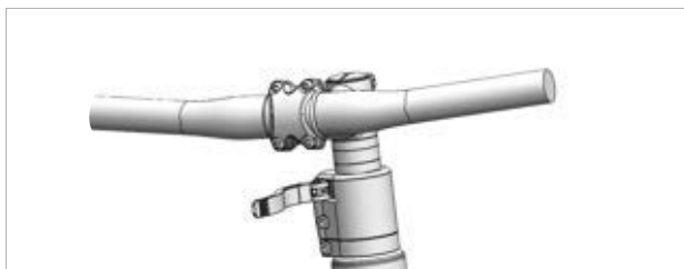
Figura 151: Esempio: All Up con leva di serraggio dell'attacco manubrio aperta
