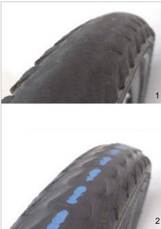
Figura 185: Pneumatico senza profilo che può essere sostituito (1) e pneumatico con protezione contro le forature in vista (2) che deve essere sostituito
