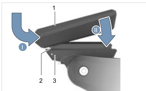
Figura 145: Montaggio del display
