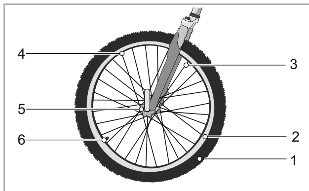
Figura 25: Componenti visibili della ruota
