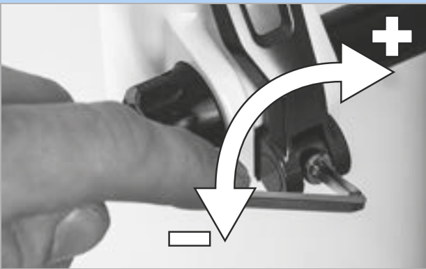
Figura 92: Regolazione della forza di serraggio del bloccaggio rapido
