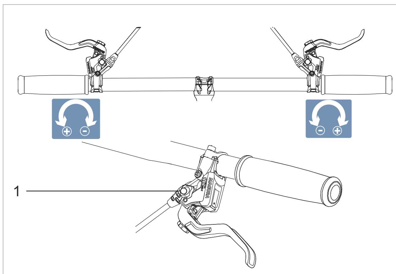
Figura 133: Uso della manopola (1) per la regolazione del punto di pressione
