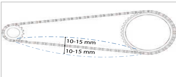
Figura 210: Controllo della tensione della catena, esempio: 5 mm verso l'alto, 10 mm verso il basso = scostamento 15 mm
