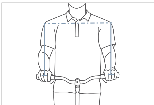
Figura 117: Individuazione della larghezza ottimale del manubrio
