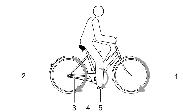
Figura 47: Schema del sistema di trazione meccanico
