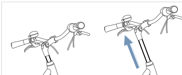
Figura 121: Regolazione dell'altezza dell'attacco manubrio a canotto
