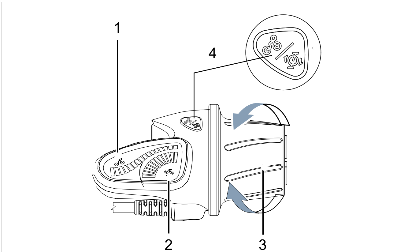
Figura 75: Manopola ENVIOLLO con indicatore
