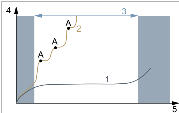
Figura 181: Diagramma dell'usura, asportazione di materiale (y) in funzione della durata di funzionamento (x)
