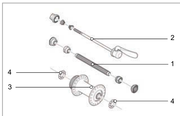
Figura 33: Esempio di mozzo della ruota anteriore, SHIMANO
