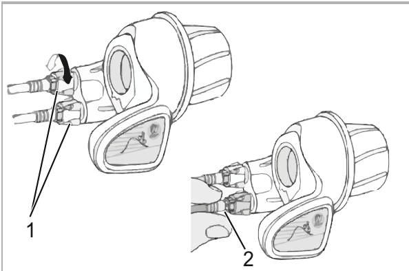
Figura 214: Interruttore a manopola con boccole di regolazione (1) con gioco angolare (2)
