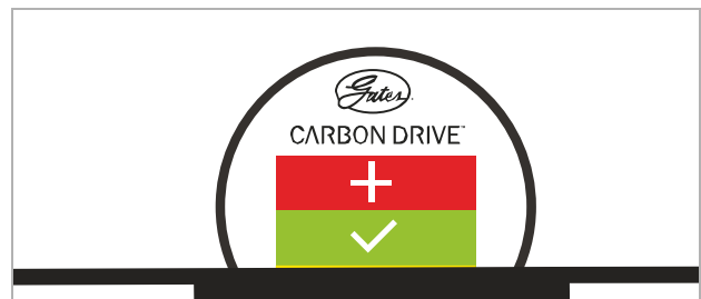
Figura 208: Esempio: indicatore sul bordo del settore giallo, per cui ridurre leggermente la tensione della cinghia
