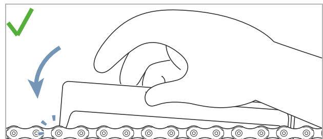
Figura 196: Il calibro di misura dell'usura non entra tra le maglie
