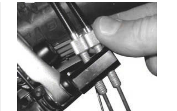
Figura 211: Le versioni del mozzo ROHLOFF con comando interno del cambio hanno i regolatori del tensionamento sul controsupporto di tensionamento
