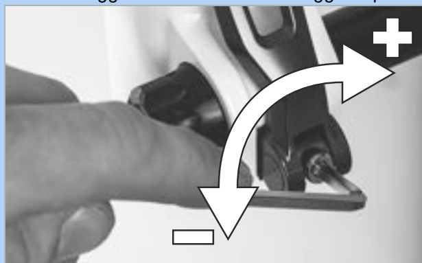
Figura 216: Regolazione della forza di serraggio del bloccaggio rapido
