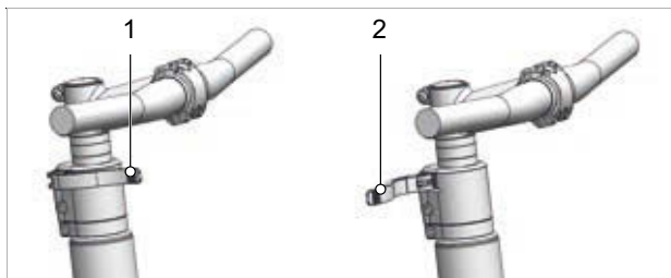
Figura 119: Leva di serraggio dell'attacco manubrio chiusa (1) e aperta (2), esempio All Up
