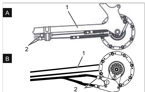
Figura 213: Boccole di regolazione (2) di due versioni alternative (A e B) di un cambio azionato da cavo doppio sul fodero orizzontale (1)
