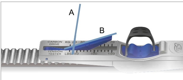
Figura 205: Esempio di lettura del valore: 20 kg
