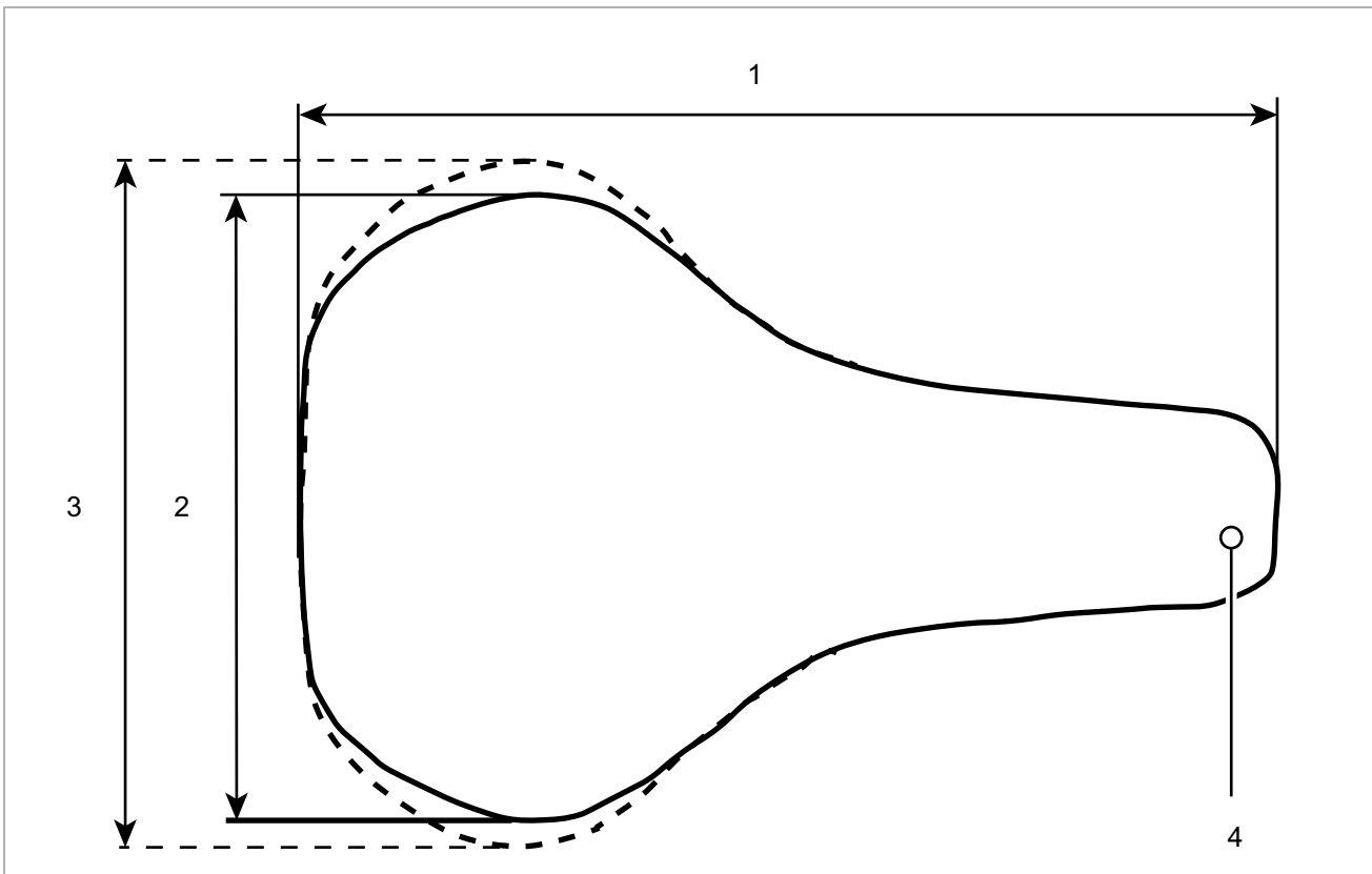
Figura 34: Dimensioni sella
