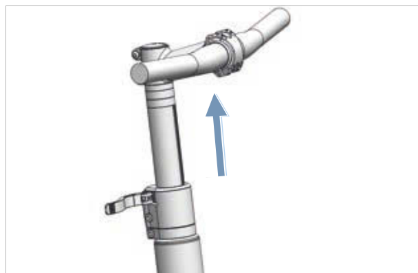
Figura 120: Sollevamento del manubrio, esempio All Up
