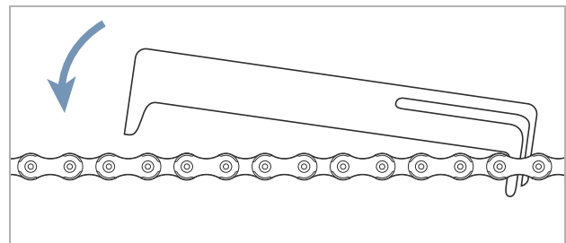
Figura 195: Abbassamento del calibro di misura dell'usura a sinistra
