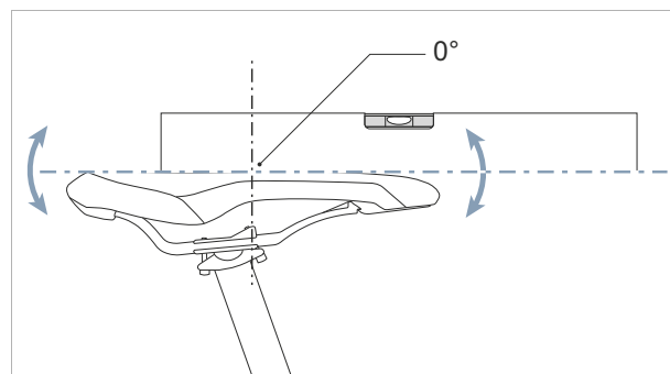
Figura 116: Sella in posizione orizzontale con angolo di inclinazione di 0° del centro della sella
