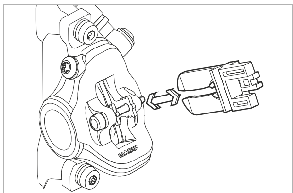
Figura 81: Fissaggio della sicura di trasporto
