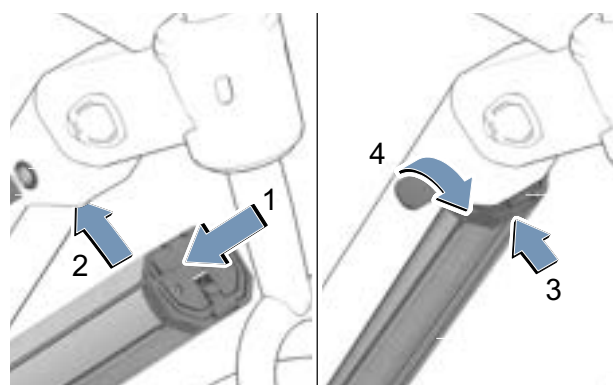
Figura 162: Montaggio della batteria integrata
