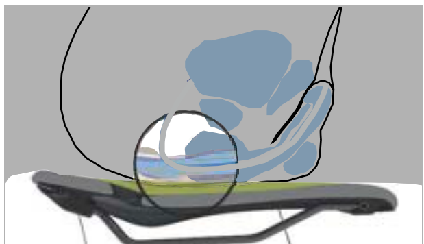
Figura 38: Punti di pressione della sella, anatomia maschile
