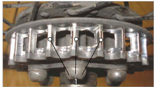
Figura 201: Esempio: profilo usurato dei denti
