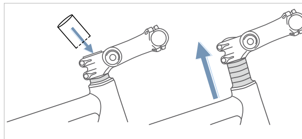
Figura 122: Aumento dell'altezza dell'attacco manubrio ahead tramite montaggio di distanziatori ad anello (spaziatori)
