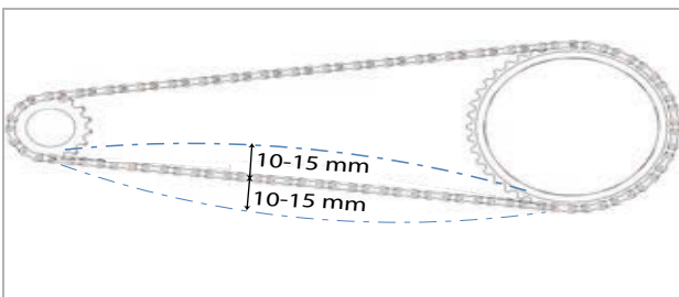
Figura 188: Controllo della tensione della catena, esempio: 5 mm verso l'alto, 10 mm verso il basso = scostamento 15 mm
