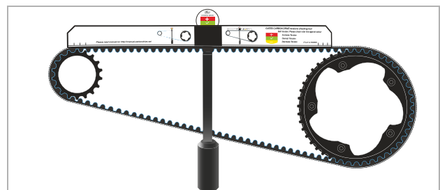
Figura 207: Righello posizionato
