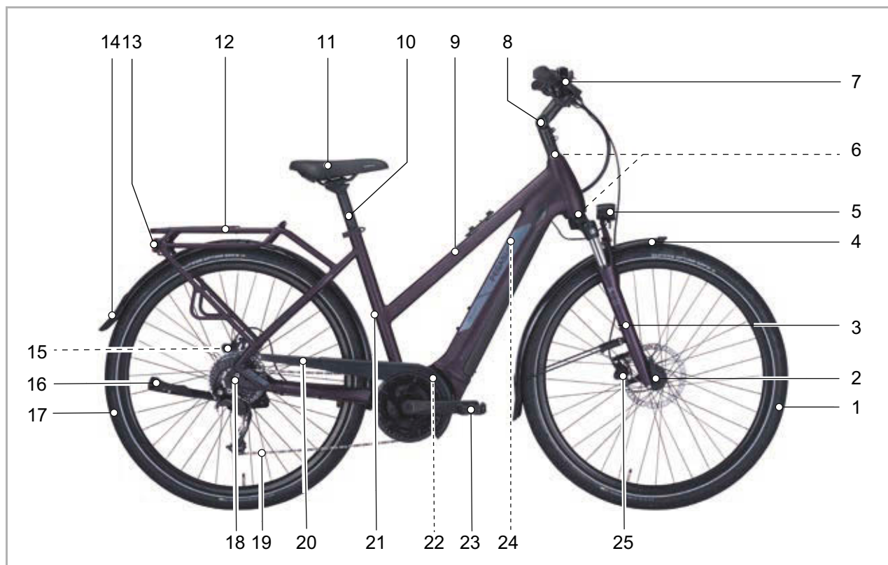
Figura 3: Vista del pedalec da destra, esempio Pegasus Solero Evo 9
