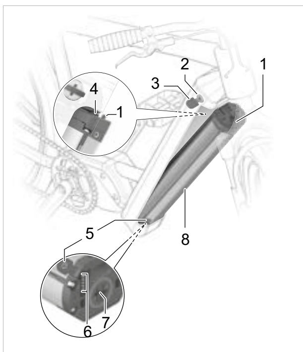
Figura 52: Dettagli PowerTube
