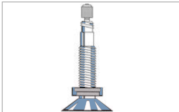
Figura 31: Valvola Presta
