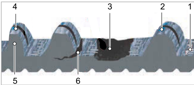
Figura 198: Caratteristiche di usura di una cinghia
