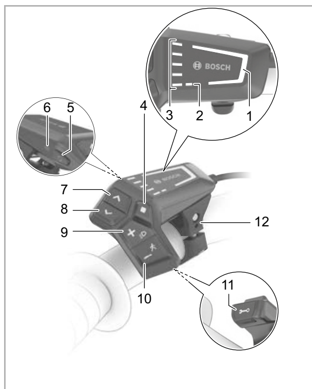
Figura 164: Schema del computer di bordo BOSCH LED Remote
