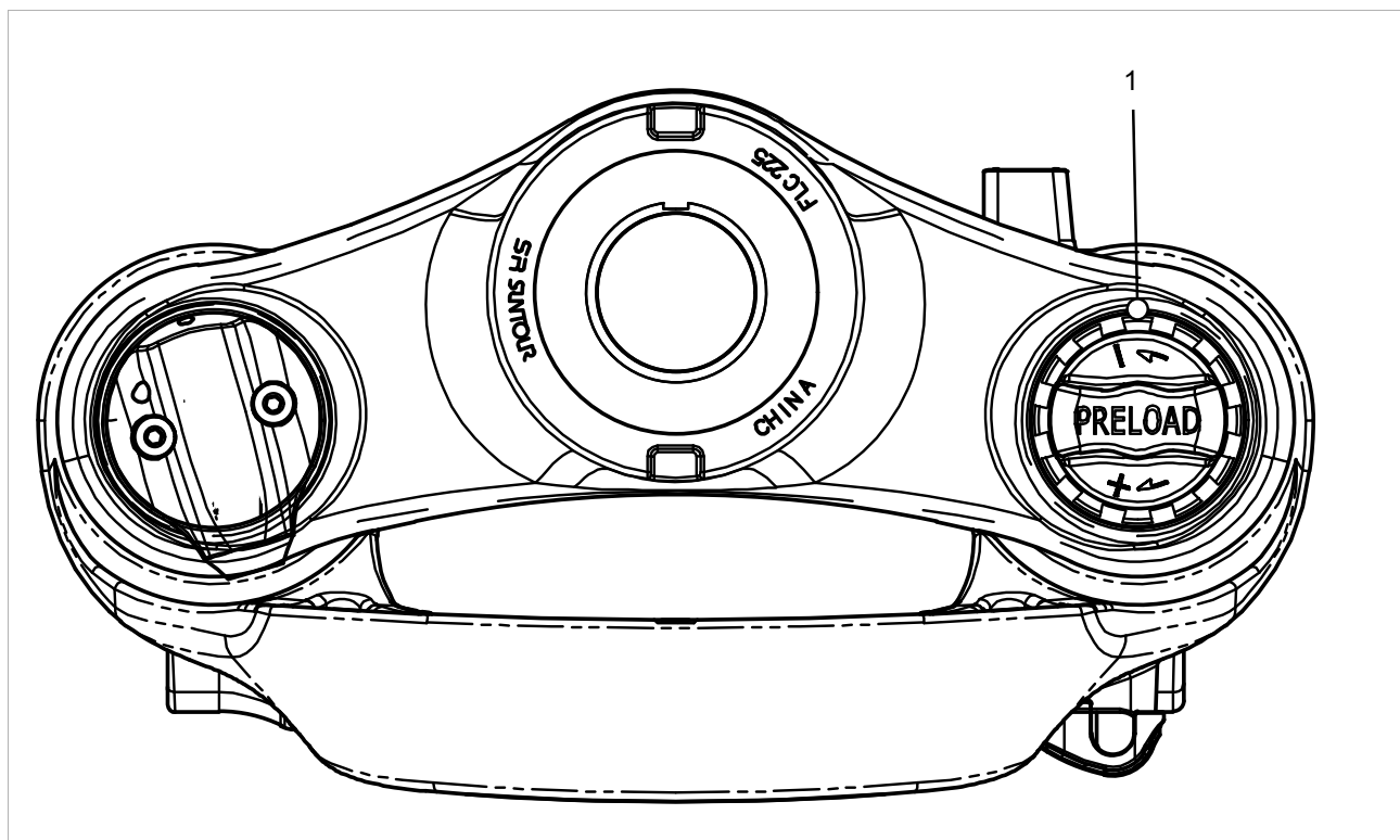
Figura 139: Esempio SR SUNTOUR, manopola di regolazione della SAG sulla corona della forcella
