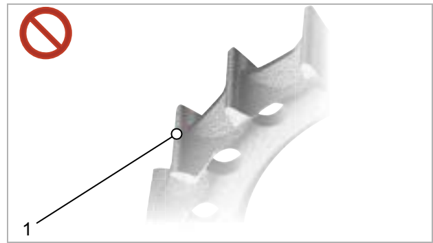
Figura 200: Profilo usurato dei denti
