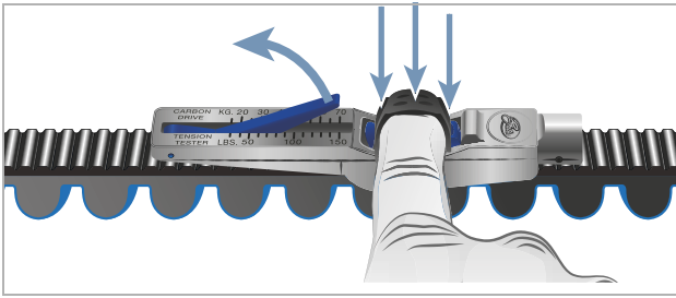
Figura 204: Spinta del calibro di verifica verso il basso con il dito
