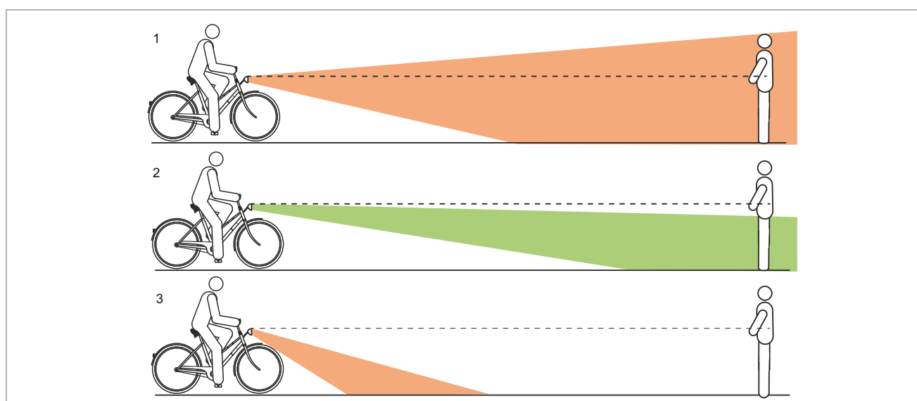
Figura 142: Luce regolata a un'altezza eccessiva (1), correttamente (2) e a un'altezza insufficiente (3)
