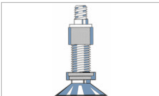
Figura 30: Valvola Dunlop
