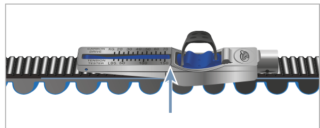
Figura 203: Calibro sulla cinghia
