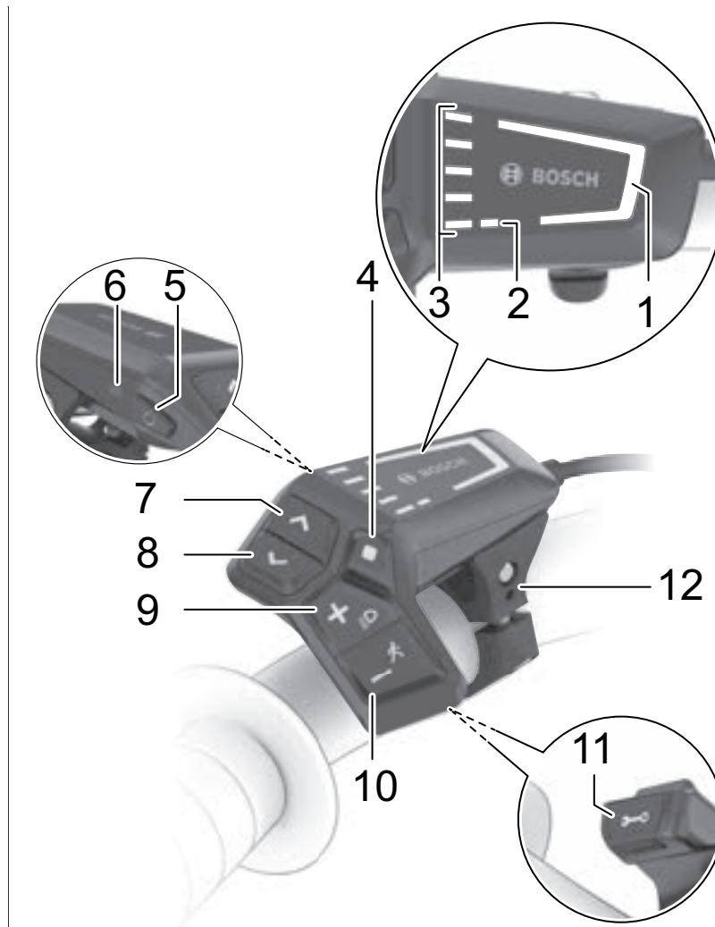
Abbildung 33: Übersicht Bedieneinheit BOSCH LCD Remote
