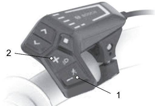
Abbildung 107: Lage Plus-Taster und Minus-Taster
