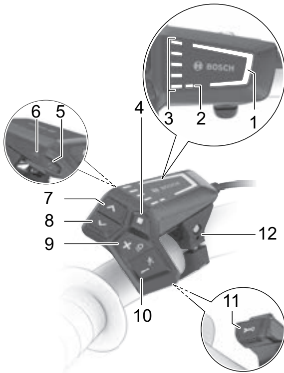
Abbildung 103: Übersicht Bedieneinheit BOSCH LCD Remote
