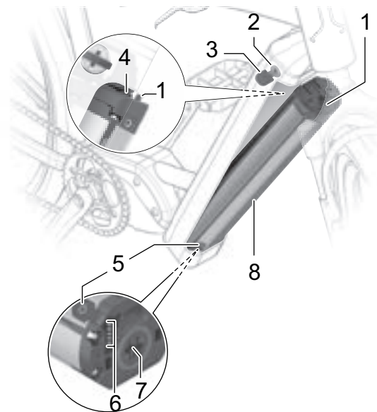
Abbildung 30: Detail PowerTube 750
