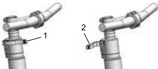
Abbildung 70: Geschlossener (1) und geöffneter (2) Vorbau-Spannhebel, Beispiel All Up
