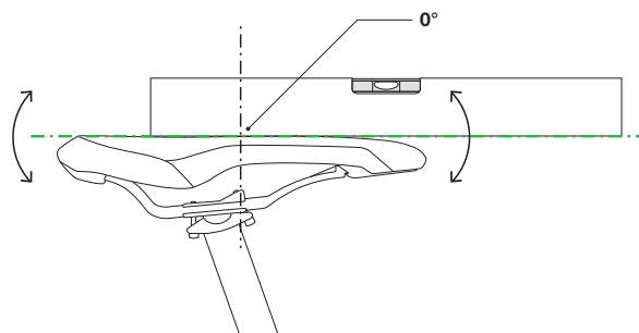
Abbildung 67: Waagerechte Sattelneigung mit 0° Neigung in der Sattelmitte
