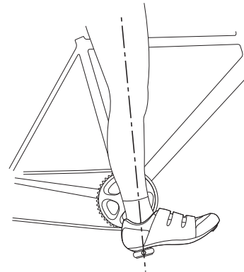
Abbildung 62: Fersenmethode
