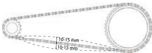
Abbildung 124: Kettenspannung prüfen
