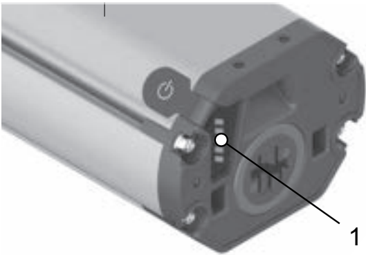
Abbildung 34: Lage Ladezustandsanzeige (Akku) (1)
