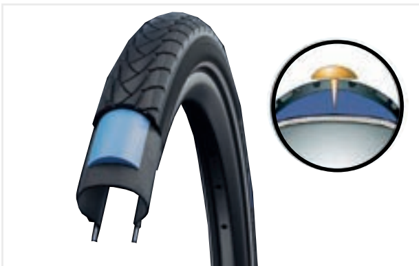
Abbildung 28: Wirkung Pannenschutz-Gürtel
