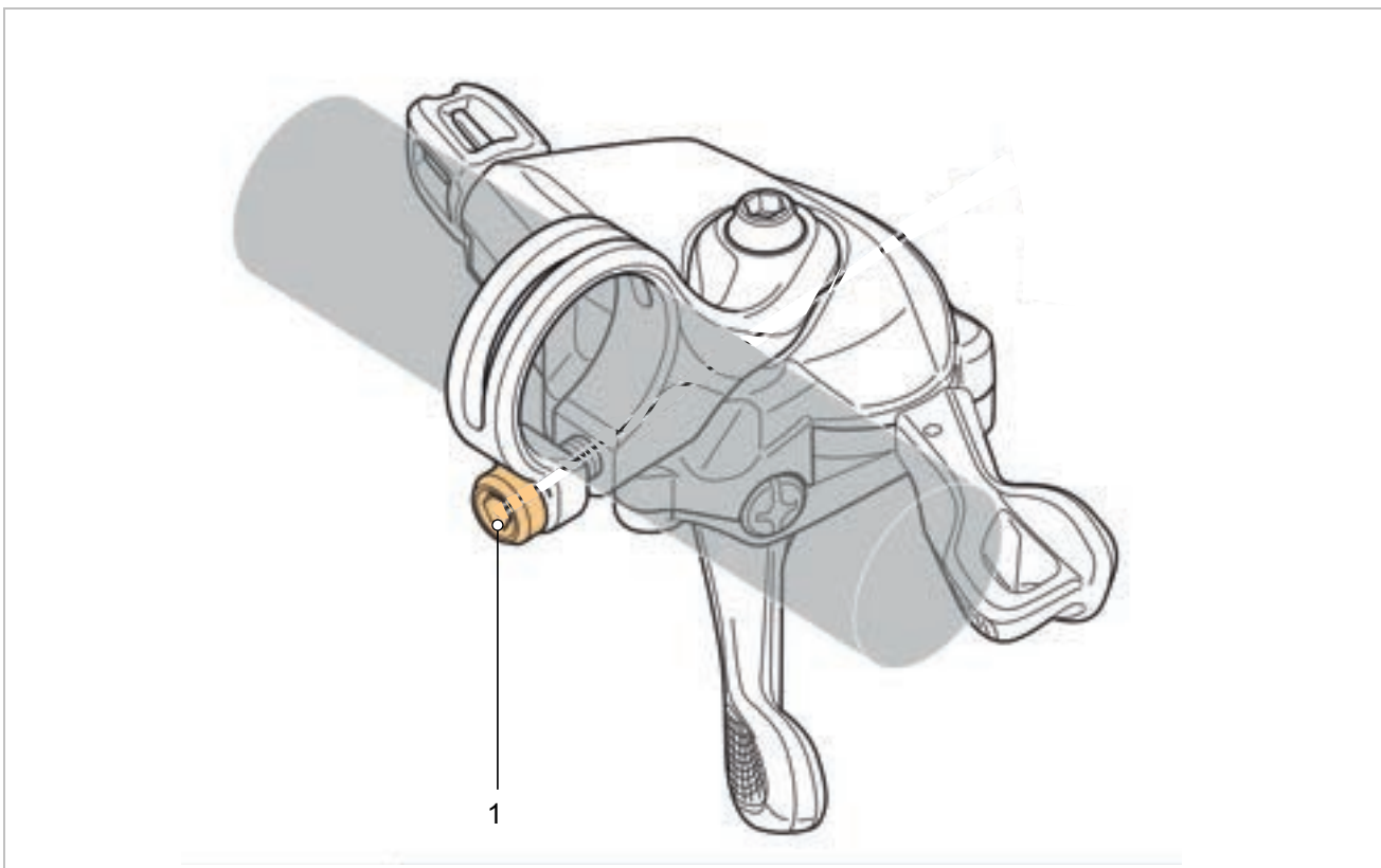
Abbildung 134: Lage Befestigungsschraube Schalthebel SHIMANO (1)
