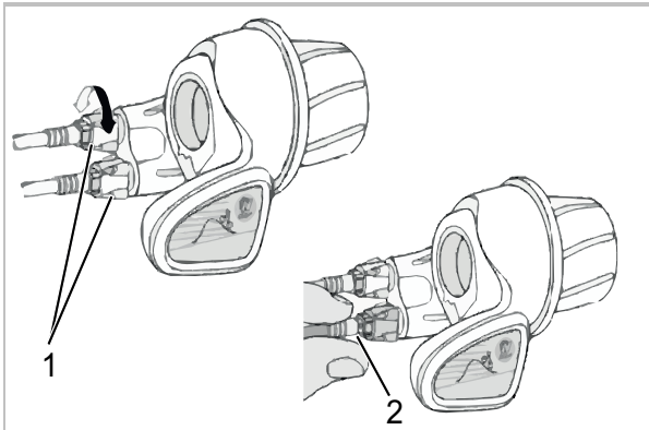
Abbildung 214: Drehgriffschalter mit Einstellhülse (1) mit Drehspiel (2)
