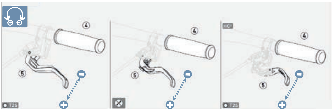
Abbildung 131: Griffweite Handbremse MAGURA Scheibenbremse einstellen
