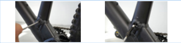
Afbeelding 178: Zadelpen loshalen
