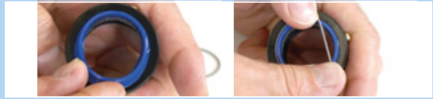
Afbeelding 189: Afstrijker inleggen en bevestigen
