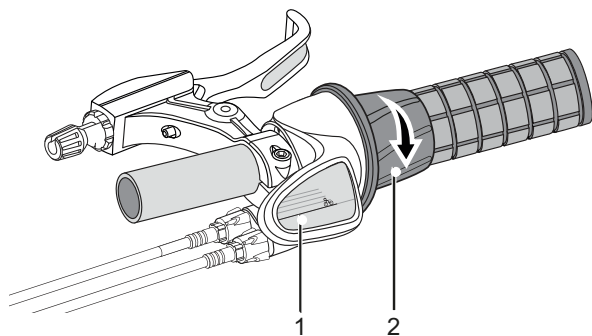
Afbeelding 43: Weergave vlakke (1) bij het omhoog schakelen (2)
