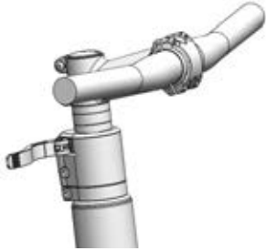
Afbeelding 120: Voorbeeld All Up met geopende voorbouwspanhendel
