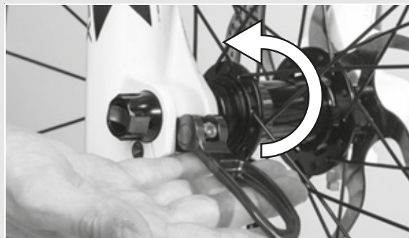
Figura 35: Bloccaggio della leva
