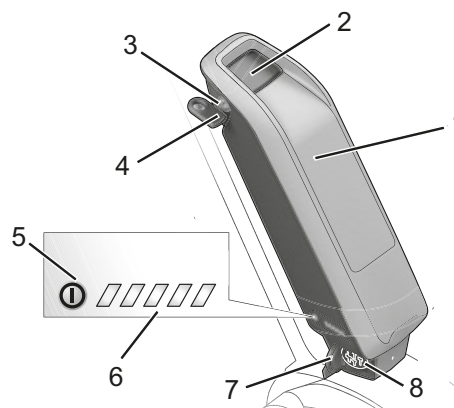
Figura 16: Dettaglio della batteria sul tubo trasversale
