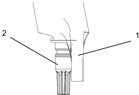
Figura 60: Regolatore del rebound Suntour (2) sulla forcella (1)
