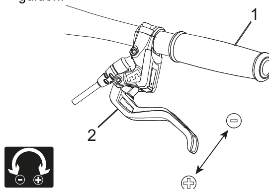
Illustration 50 : Utilisation de la vis de réglage (2) pour ajuster la distance entre le levier de frein et la poignée de guidon (1)
