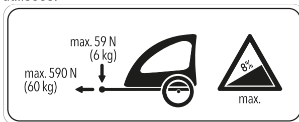
Illustration 60 : Plaque d'information de la remorque
