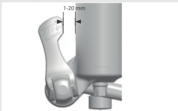
Illustration 37 : Distance entre levier et montant de fourche
