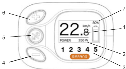
Illustration 18 : Aperçu de la structure et des éléments de commande de l'écran
