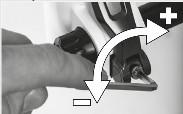
Illustration 31 : Régler la force de serrage de l'attache rapide
