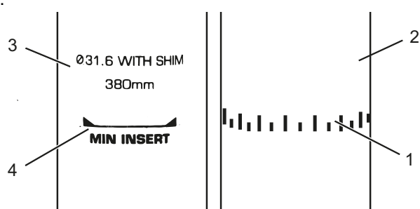
Illustration 43 : Vue détaillée de la tige de selle, exemples de marquage de la profondeur d'insertion minimale
