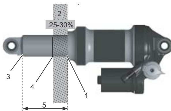
Illustration 58 : Structure d'un amortisseur arrière FOX
