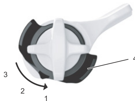
Illustration 79 : Le réglage fin de la position OUVERT se fait au moyen du dispositif de réglage (4)
