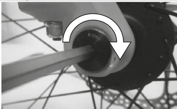
Illustration 21 : Serrer l'axe
