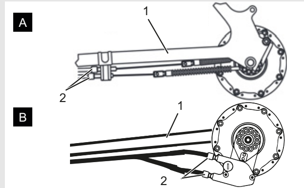
Illustration 87 : Douilles de réglage (2) sur deux modèles alternatifs (A et B) d'un changement de vitesse actionné par câble à deux câbles sur la base de cadre (1)
