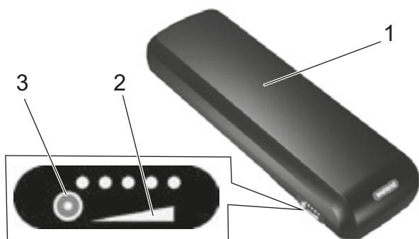
Illustration 17 : Détail de la batterie pour tube inférieur ou tube de selle
