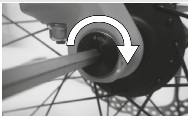
Illustration 12 : Serrer l'axe
