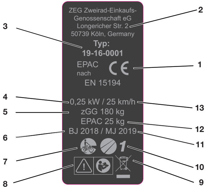
Plaque signalétique, exemple
