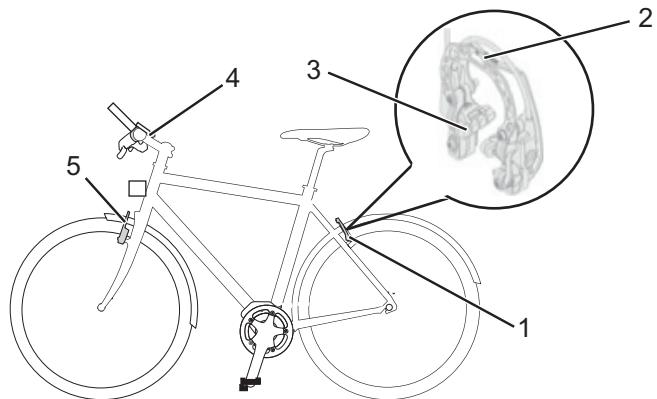
Illustration 7 : Composants du frein de jante avec détails, exemple d'un Magura HS22
