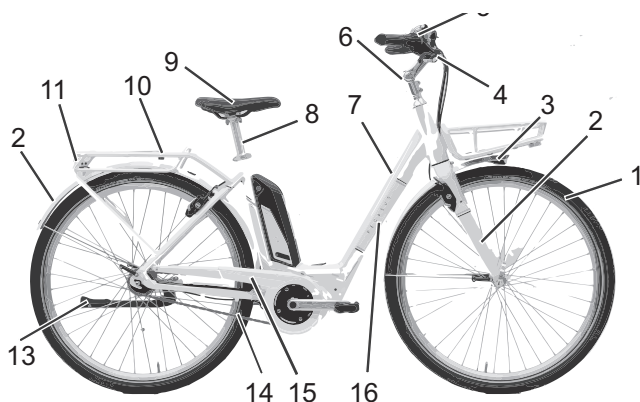
Vélo vu de droite, exemple d'un Comfort 5 Belt
