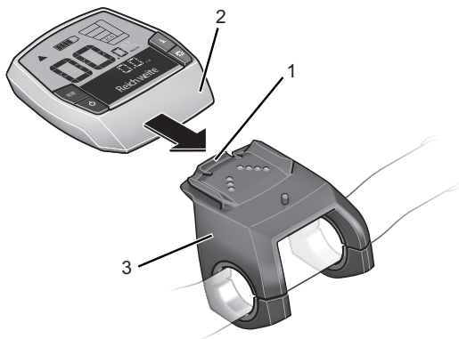
Illustration 54 : Enfoncer l'écran (2) via le dispositif de blocage de l'écran (1) jusqu'à la butée du support (3)
