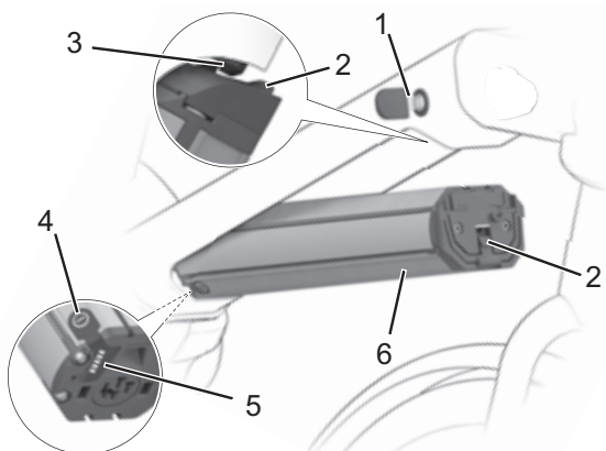
Illustration 14 : Détail de la batterie intégrée
