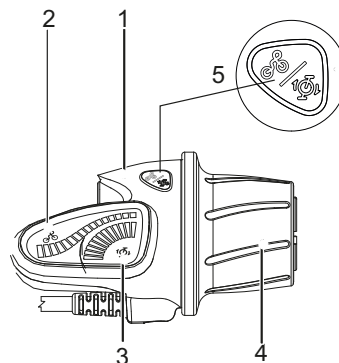
Afbeelding 82: enviolo draaibaar handvat met weergave
