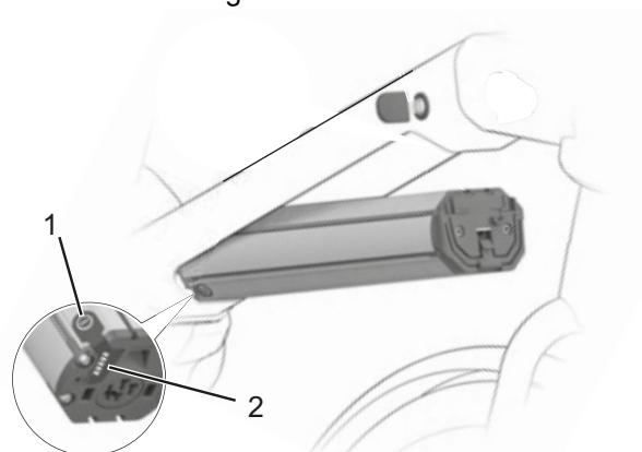
Afbeelding 20: Voorbeeld laadtoestandweergave
