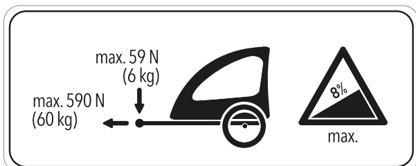
Afbeelding 67: Waarschuingssticker aanhanger
