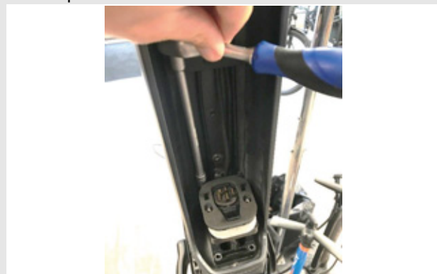
Afbeelding 24: Binnenzeskantschroeven verwijderen
