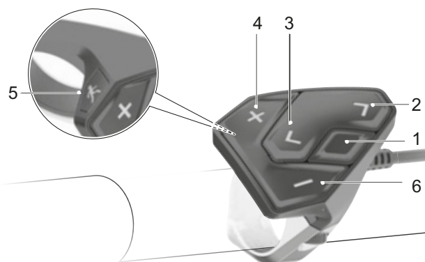
Afbeelding 18: Overzicht bedieningselementen
