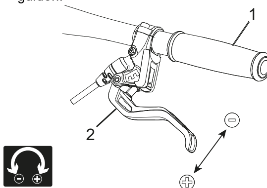
Illustration 52 : Utilisation de la vis de réglage (2) pour ajuster la distance entre le levier de frein et la poignée de guidon (1)
