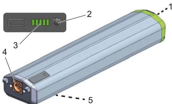
Illustration 16 : Détail d'une batterie intégrée
