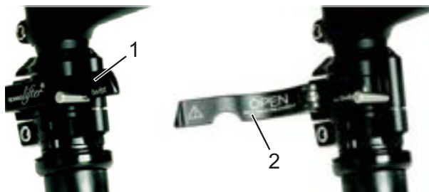
Illustration 48 : Levier de serrage fermé (1) et ouvert (2) sur la potence, exemple d'un by.schulz speedlifter
