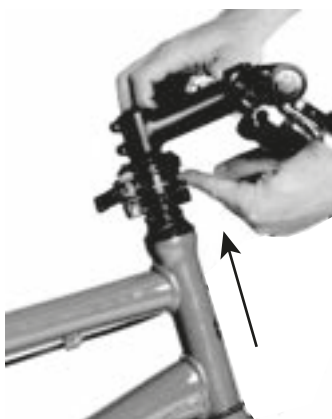
Illustration 49 : Tirer le levier de blocage vers le haut, exemple d'un by.schulz speedlifter
