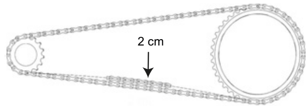
Illustration 70 : Contrôler la tension de la chaîne
