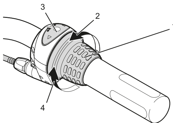
Illustration 69 : Exemple d'un changement de vitesse Shimano Nexus : Poignée de vitesse rotative (1) du moyeu à vitesses intégrées avec son affichage (3), le sens de rotation pour passer à une vitesse supérieure (2) et le sens de rotation pour une vitesse inférieure (4)
