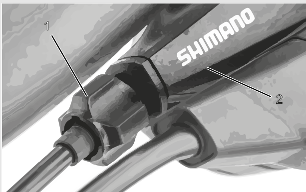
Illustration 73 : Douille de réglage (1) du changement de vitesse à un câble actionné par câble avec boîtier de manette de vitesse (2), exemple
