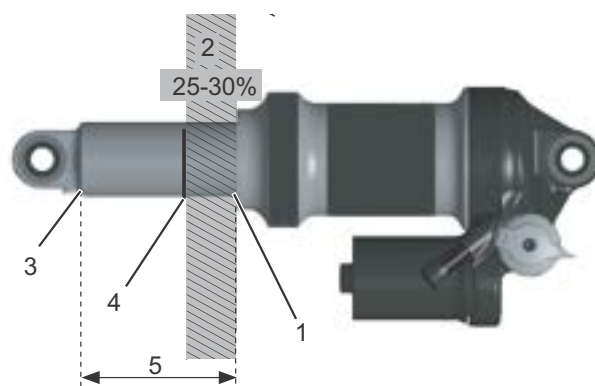
Illustration 60 : Structure d'un amortisseur arrière FOX
