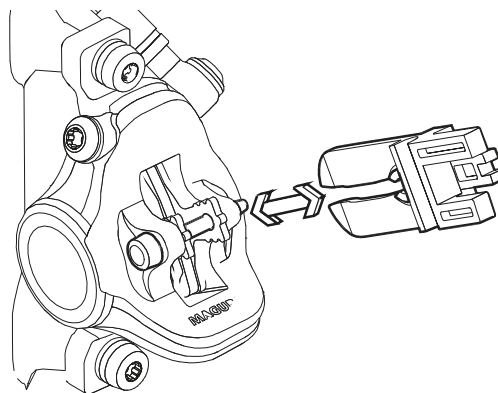
Illustration 21 : Fixer la sécurité de transport
