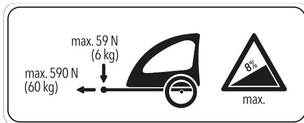
Illustration 62 : Plaque d'information de la remorque
