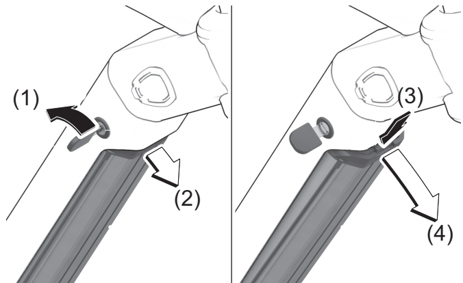
Abbildung 51: Integrierte Batterie herausnehmen
