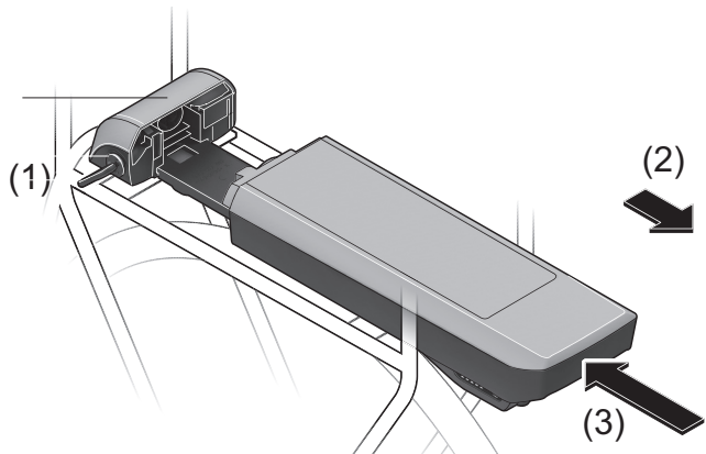
Abbildung 50: Gepäckträgerbatterie herausnehmen und einsetzen
