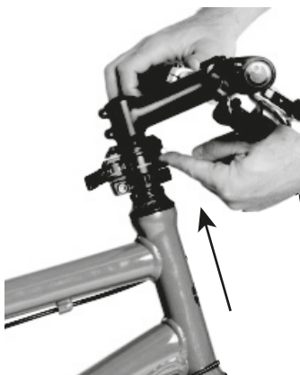
Figura 38: Sollevamento della leva di sicurezza, esempio by.schulz speedlifter
