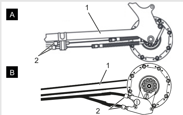
Figura 57: Boccole di regolazione (2) di due versioni alternative (A e B) di un cambio azionato da cavo doppio sul foderò orizzontale (1)
