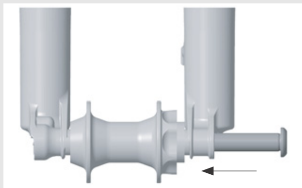
Figura 30: Inserimento dell'asse Kabolt
