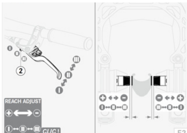
Figura 40: Regolazione dell'ampiezza di presa della leva del freno Magura HS33
