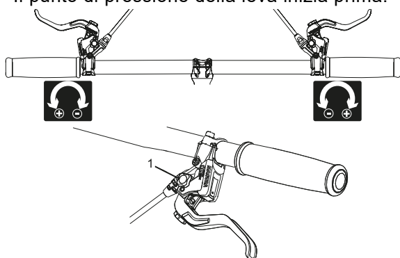
Figura 42: Uso della manopola (1) per la regolazione del punto di pressione
