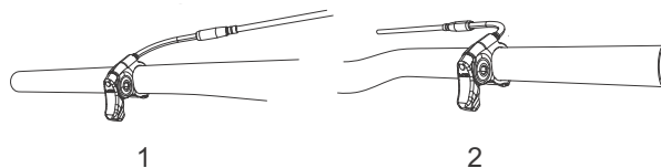
Figura 35: Leva del canotto reggisella montata a sinistra (1) o a destra (2) sul manubrio
