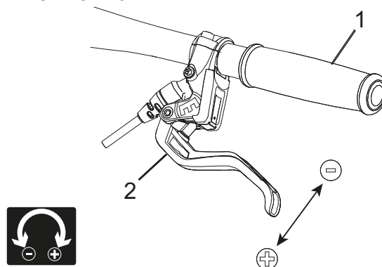
Figura 39: Regolazione dell'ampiezza di presa della leva del freno Magura HS33
