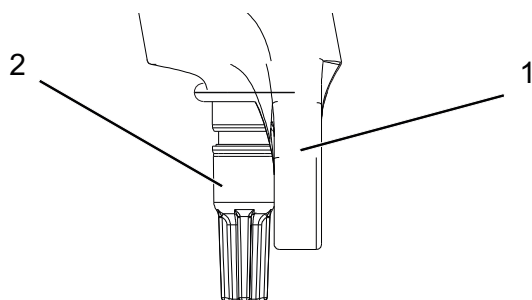
Figura 45: Vite del rebound Suntour (2), forcella (1)
