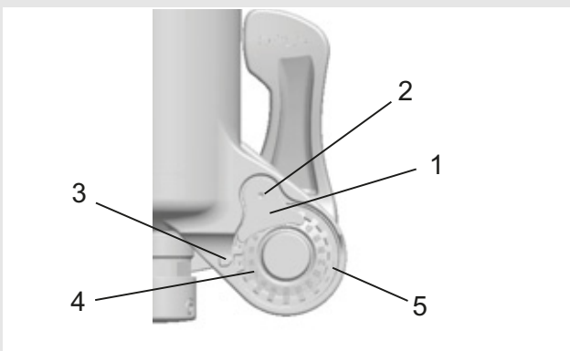
Figura 29: Vista posteriore della struttura del bloccaggio rapido con sicura del dado dell'asse (1) e dado dell'asse (5)
