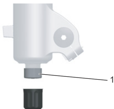
Figura 46: Regolatore del rebound FOX (1) sul forcellino della forcella
