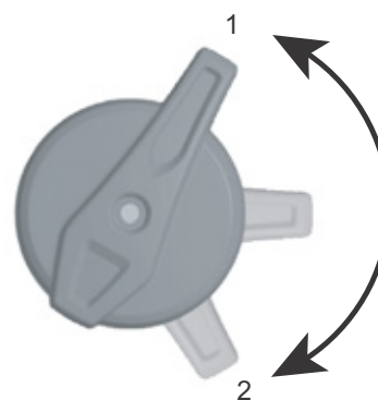
Figura 50: Regolatore dello stadio di pressione FOX con le posizioni APERTO (1) e RIGIDO (2)
