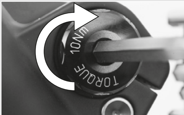
Figura 15: Serraggio dell'albero inserito
