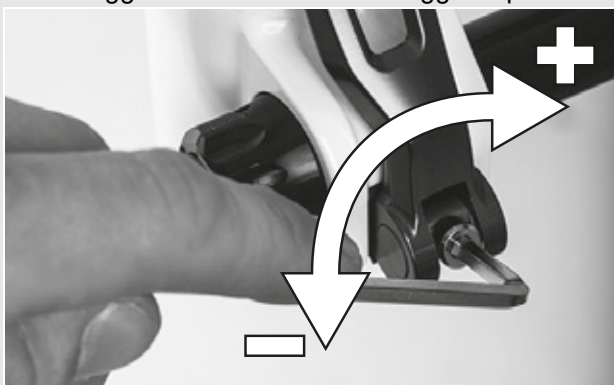
Figura 22: Regolazione della forza di serraggio del bloccaggio rapido
