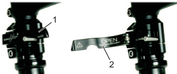
Figura 37: Leva di serraggio dell'attacco manubrio chiusa (1) e aperta (2), esempio by.schulz speedlifter
