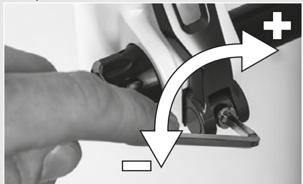
Figura 55: Regolazione della forza di serraggio del bloccaggio rapido
