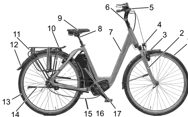
Vélo vu de droite, exemple d'un Fano E5
