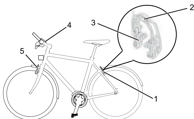
Illustration 5 : Composants du frein de jante avec détails, exemple d'un Magura HS22
