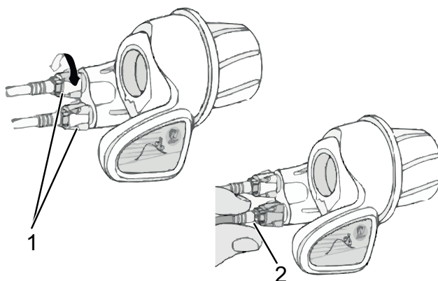
Illustration 64 : Poignée de vitesse rotative avec douilles de réglage (1) et jeu du changement de vitesse (2)
