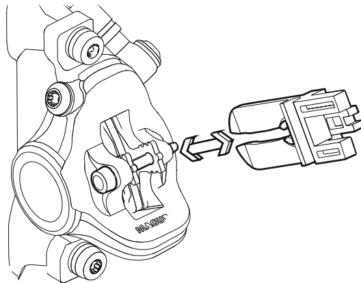
Illustration 16 : Fixer la sécurité de transport
