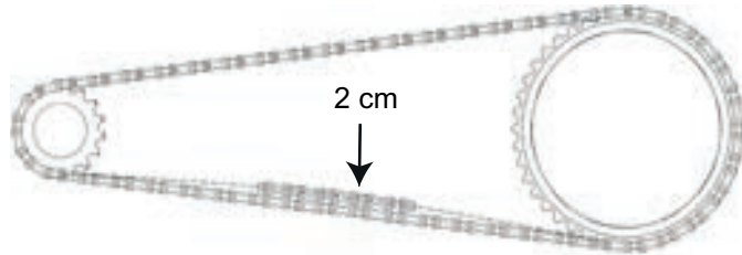
Illustration 51 : Contrôler la tension de la chaîne ou courroie
