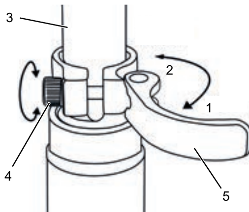
Illustration 35 : Attache rapide de la tige de selle (3) avec levier de serrage (5) et vis de réglage (4) en position ouverte (1) et sens de la position fermée (2)
