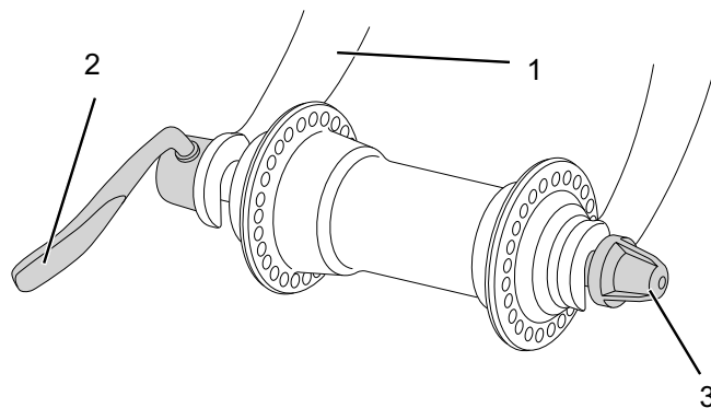
Illustration 52 : Attache rapide de la roue, modèle I, avec levier de serrage (2), fourche (1) et écrou de réglage (3)
