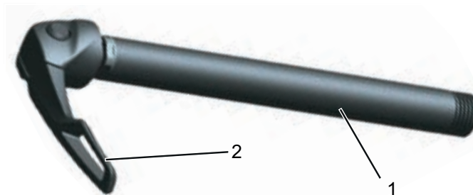
Illustration 54 : Attache rapide, modèle III, avec axe (1) et levier de serrage (2)
