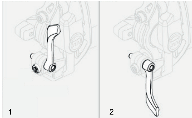
Levier de verrouillage du frein de jante, fermé (1) et ouvert (2)
