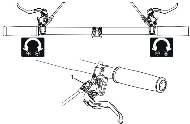
Illustration 41 : Utilisation du bouton rotatif (1) pour le réglage du point de pression
