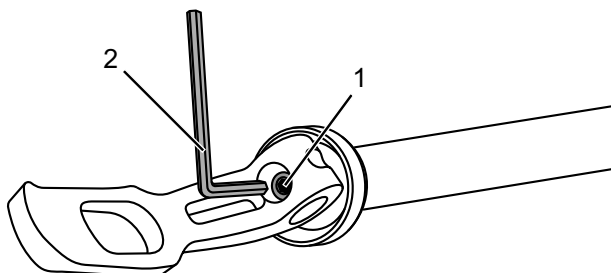
Illustration 58 : Régler la force de serrage au centre du levier de serrage (1) à l'aide d'une clé Allen (2)
